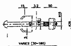
BOLT & NUT SCALE 1 : 3
