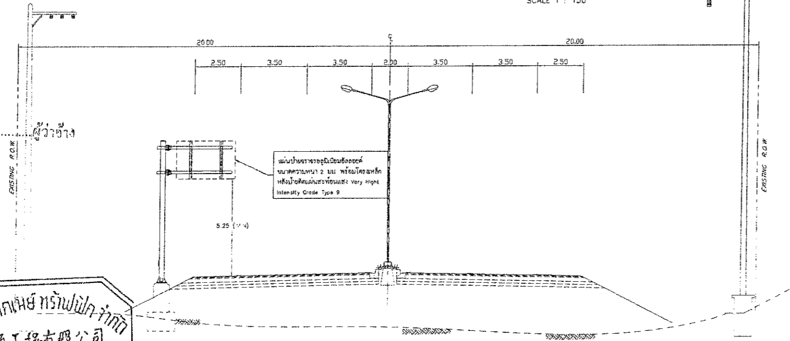
TYPICAL CROSS SECTION พท.4024 กม.0+200 LT. 0+600 LT. (หลังดำเนินการ) SCALE 1 : 150
