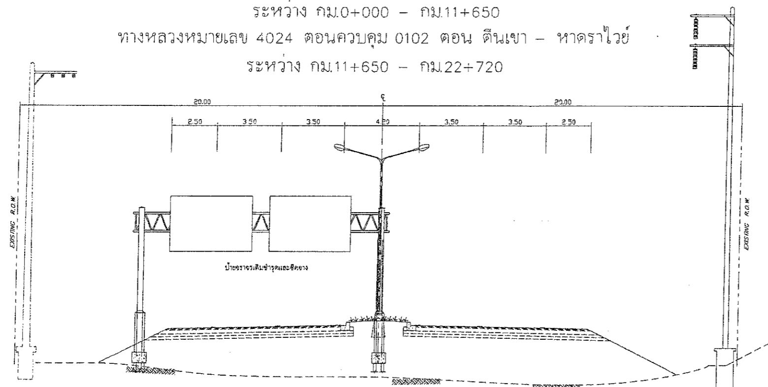
TYPICAL CROSS SECTION ทล.4024 กม.0+150 RT. (ก่อนดำเนินการ) SCALE 1 : 150
