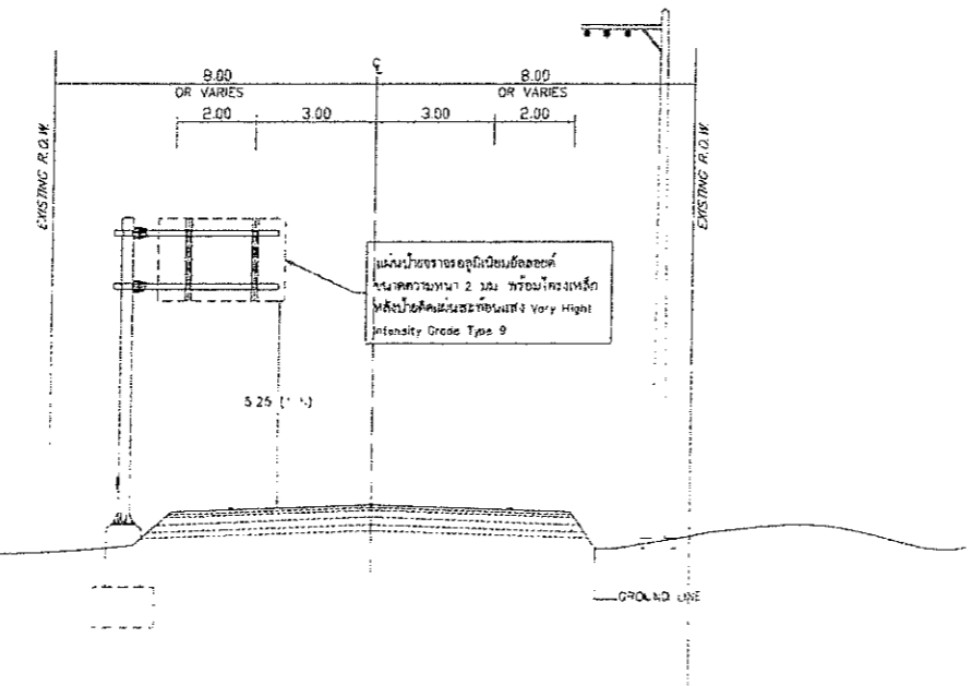
TYPICAL CROSS SECTION 4024 กม.15+400 LT. (หลังดำเนินการ) SCALE 1 : 150
