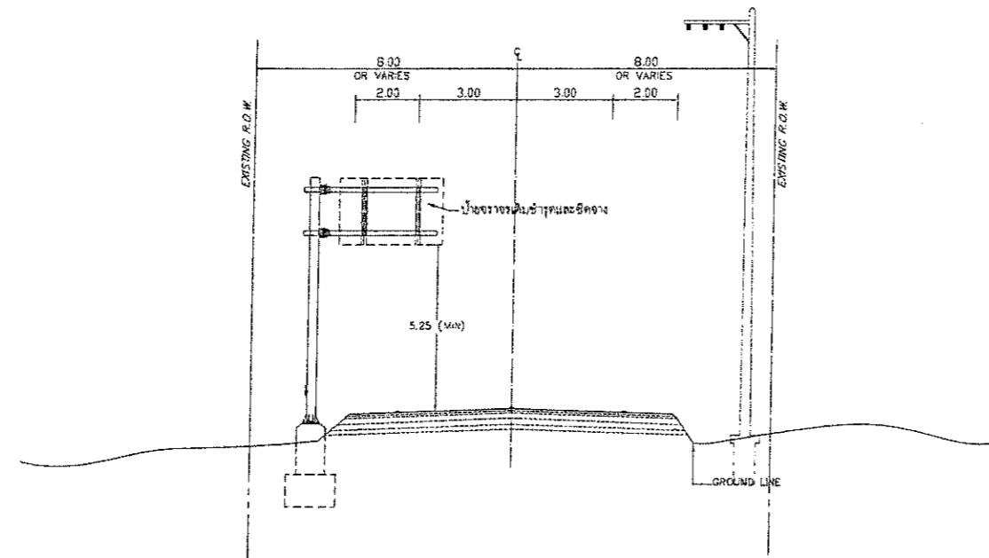
TYPICAL CROSS SECTION 4024 กม.15+400 LT. (ก่อนดำเนินการ) SCALE 1 : 150
