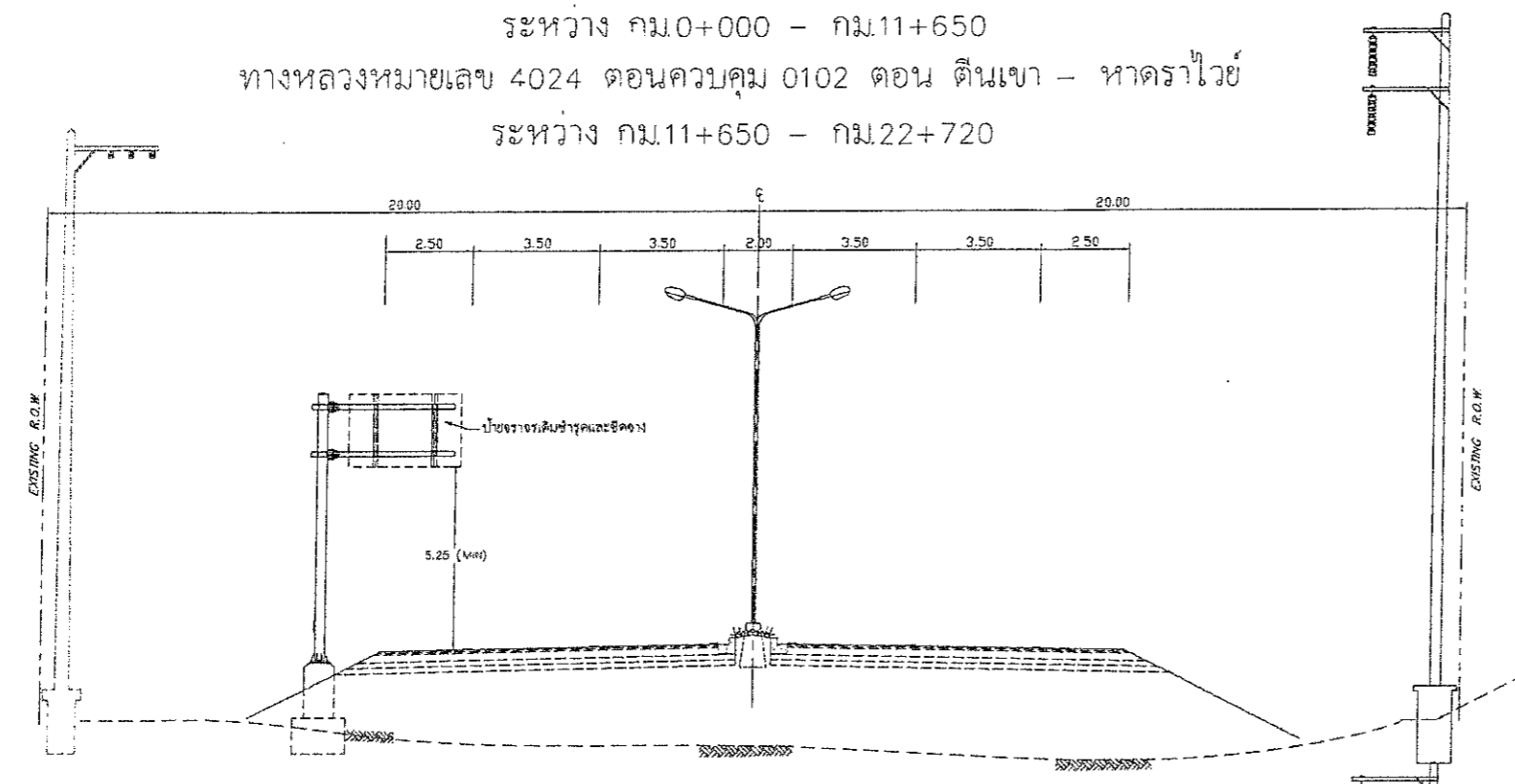
TYPICAL CROSS SECTION พท.4024 กม.0+200 LT. 0+600 LT. (ก่อนดำเนินการ) SCALE 1 : 150
