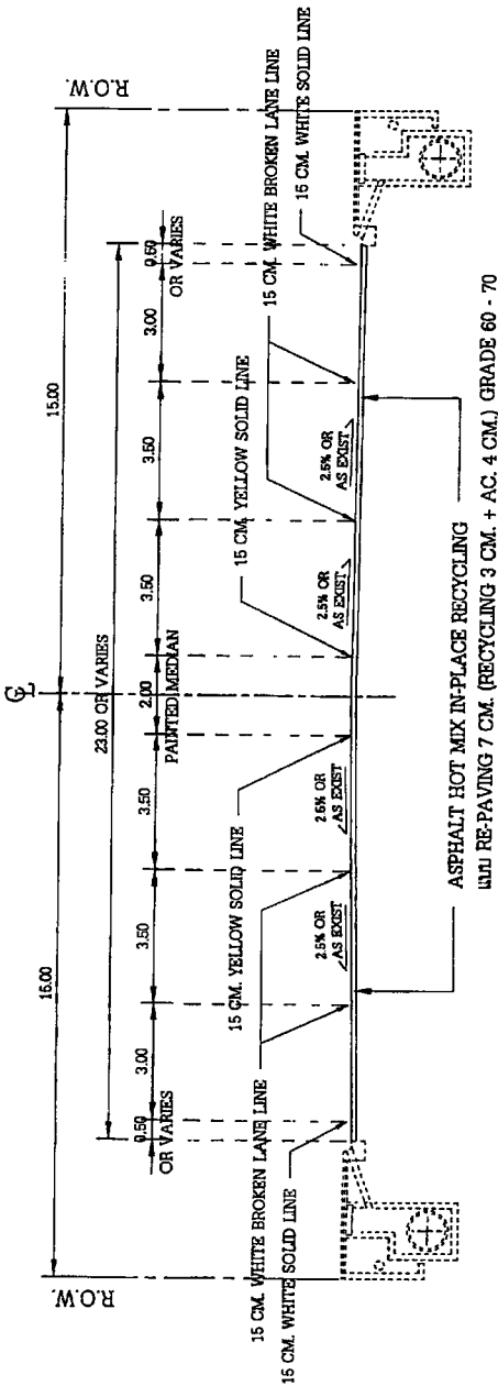
EXISTING CROSS SECTION STA. 64+300 - STA. 65+000
