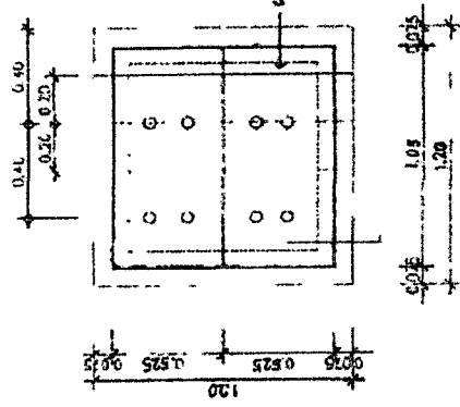
แปลนบ่อพัก มาตราส่วน 1:25
