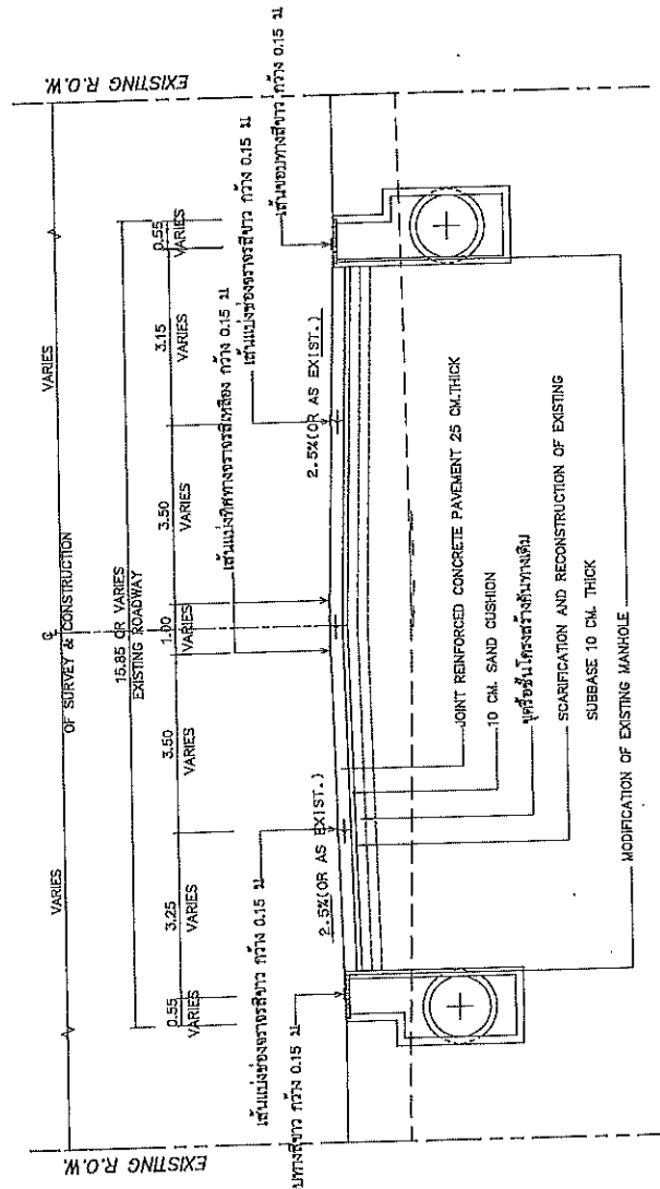
TYPICAL CROSS SECTION ระหว่าง กม.296+785 - กม.297+037 NOT TO SCALE
