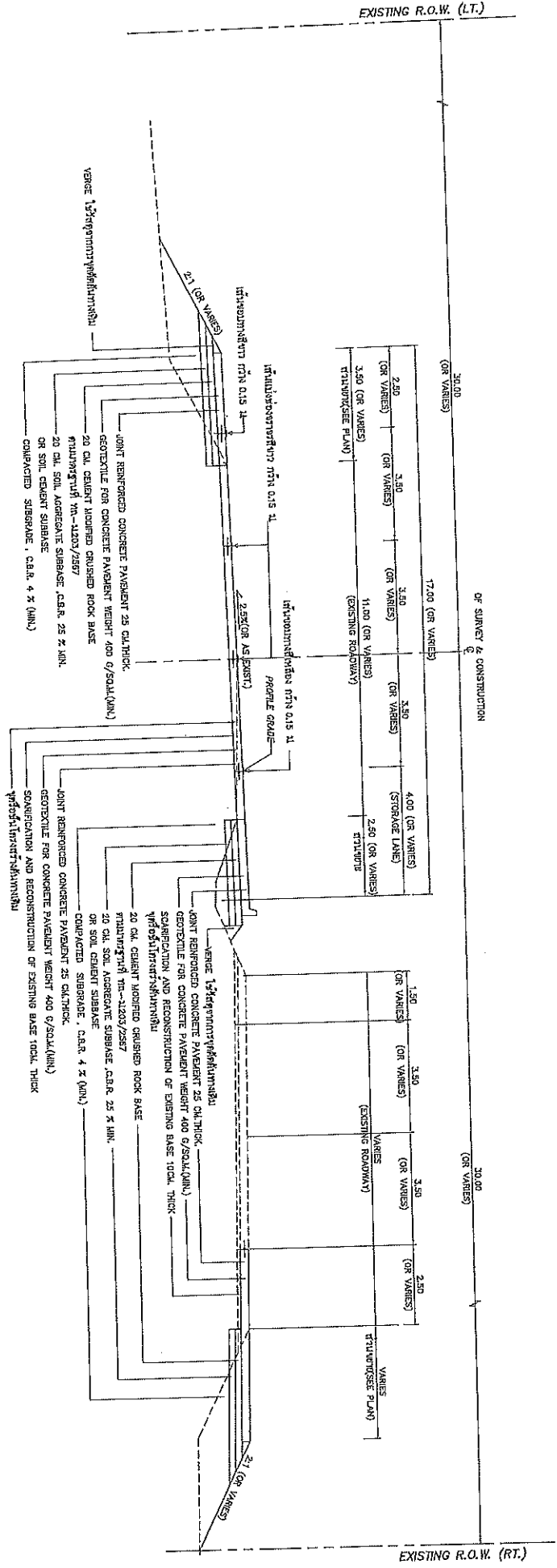
TYPICAL CROSS SECTION RM.250+370 - RM.250+600 LT., RT. (โดยโครงการ 10) NOT TO SCALE
