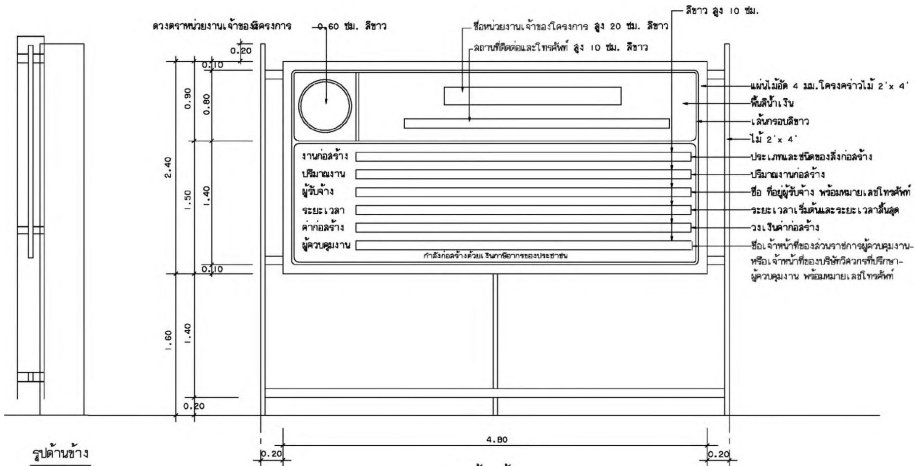
รูปด้านหน้า มาตราส่วน 1:40
