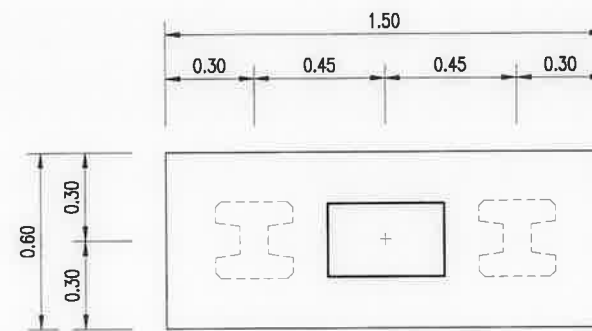
แปลนขยายฐานราก F2 SCALE 1:25
