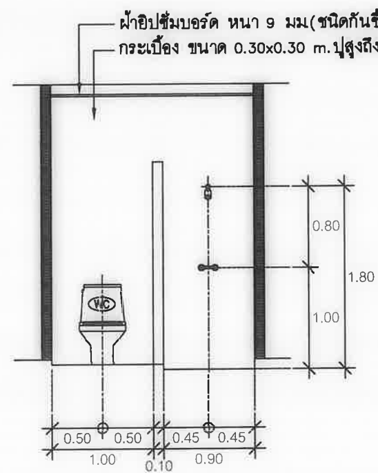
รูปตัด 7 มาตราส่วน 1:50
