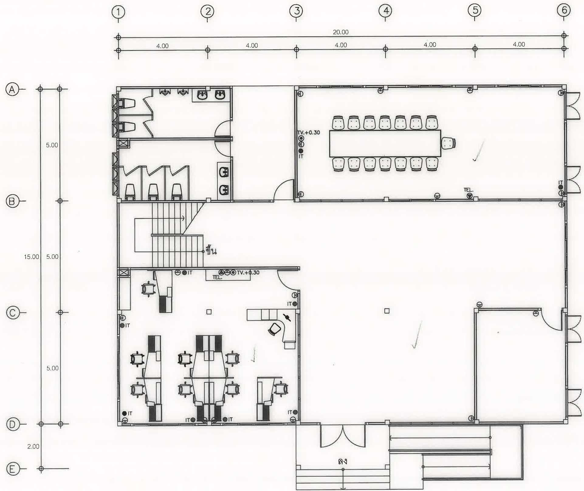
แปลนสวิตช์และปลั๊กชั้น 1 มาตราส่วน 1 : 100
