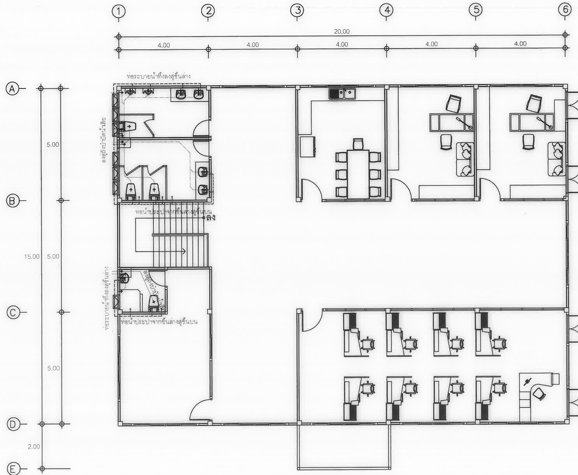
แปลนสถาปัตยกรรมชั้น 2 มาตราส่วน 1 : 100
