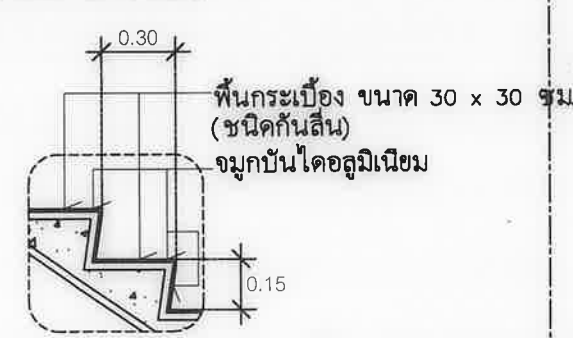
แบบขยายขึ้นบันได มาตราส่วน 1:25
