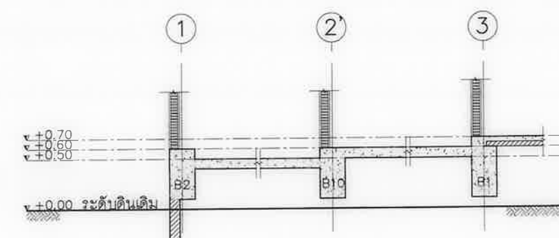
รูปตัด 1-1 มาตราส่วน 1:50
