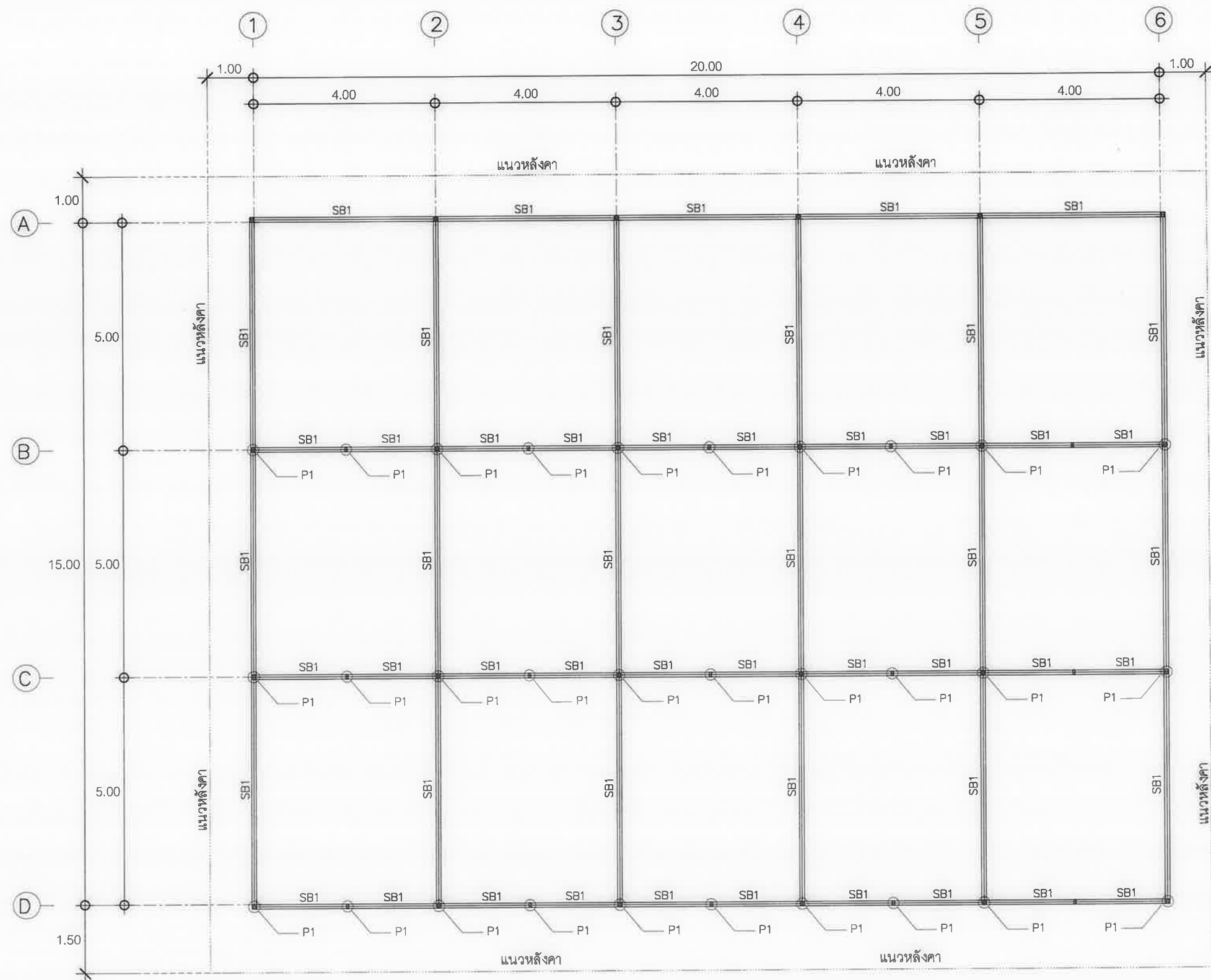
แบบแปลนอะเสเหล็ก
