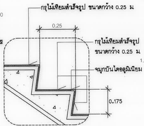
แบบขยายชั้นบันได มาตราส่วน 1:25
