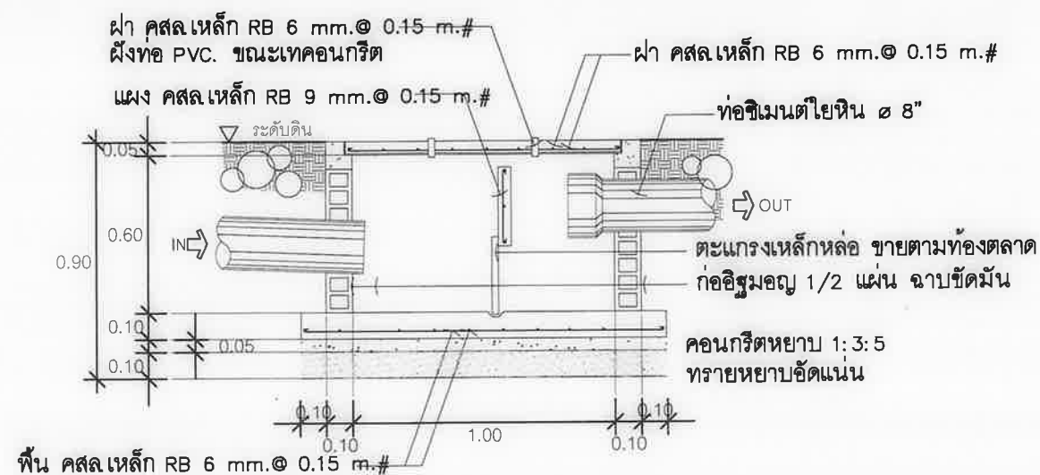
รูปตัดขยายบ่อดักขยะ-ไขมัน มาตราส่วน 1 : 25
