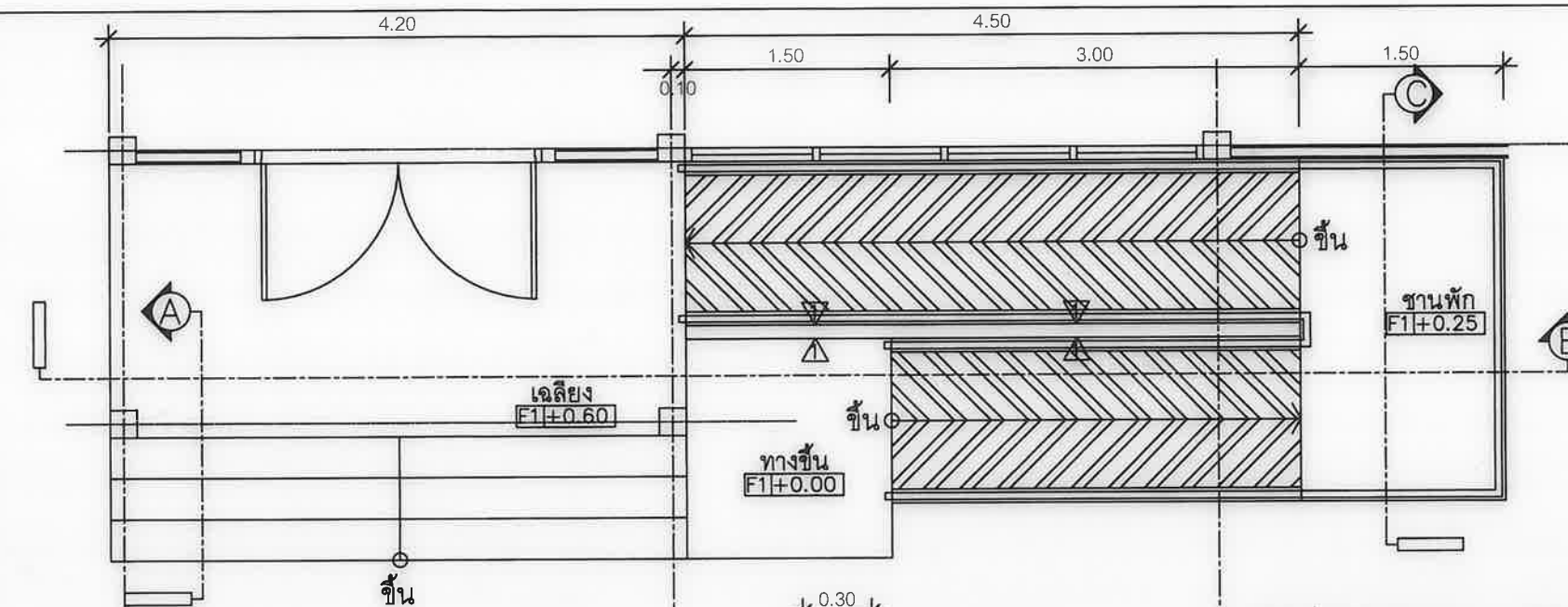
① แปลนบันได-ทางลาด ST-2 มาตราส่วน 1:50
