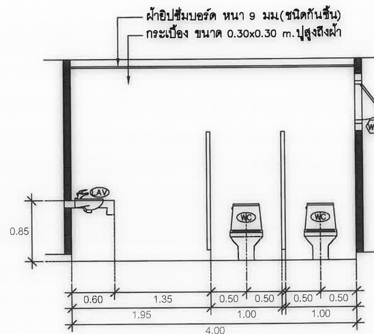
รูปตัด 5 มาตราส่วน 1:50
