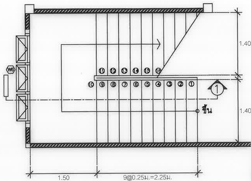
ขยายแปลนบันไดชั้น 1 มาตราส่วน 1:50
