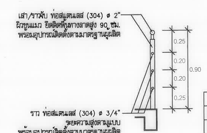
แบบขยายราวจับทางลาด มาตราส่วน 1:25
