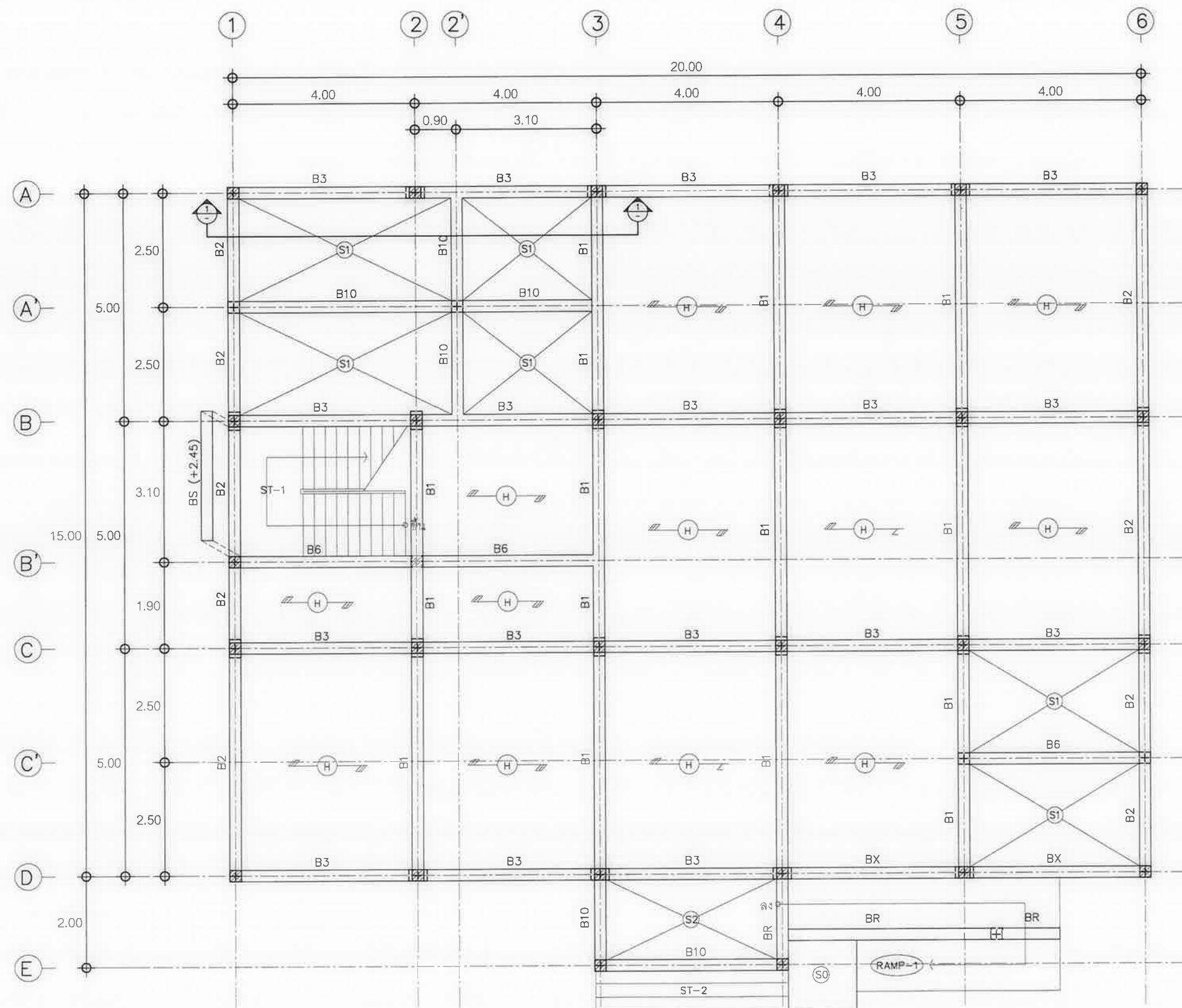
แบบแปลนคานและพื้นชั้น 1 มาตราส่วน 1:100
