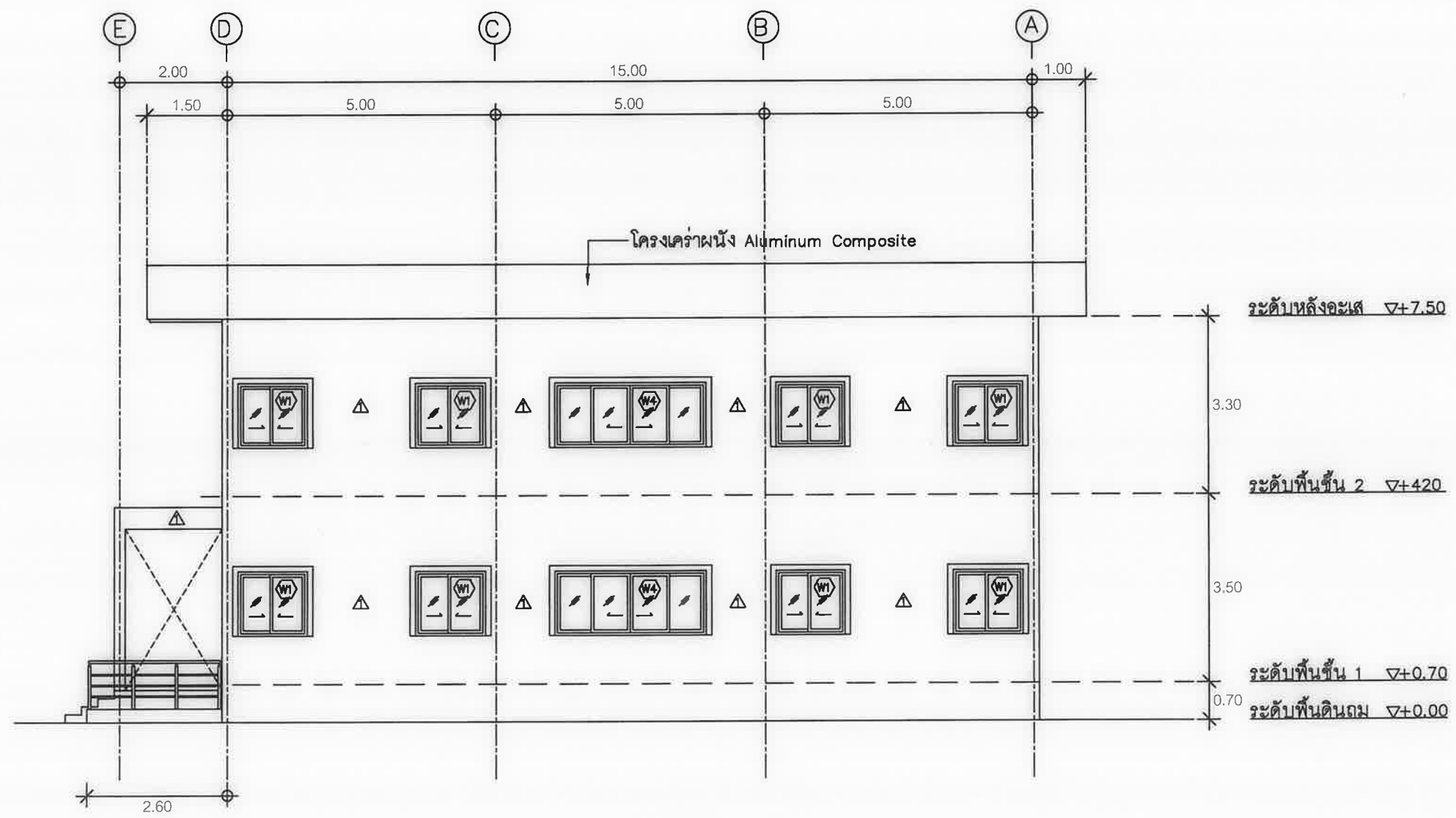
รูปด้าน 4 มาตรฐาน 1 : 100
