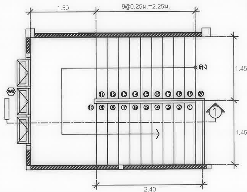
แบบขยายชั้นบันได มาตราส่วน 1:25
