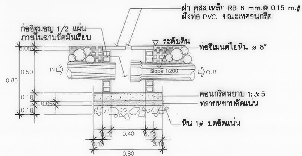
รูปตัดขยายบ่อพักน้ำทิ้ง มาตราส่วน 1 : 25
