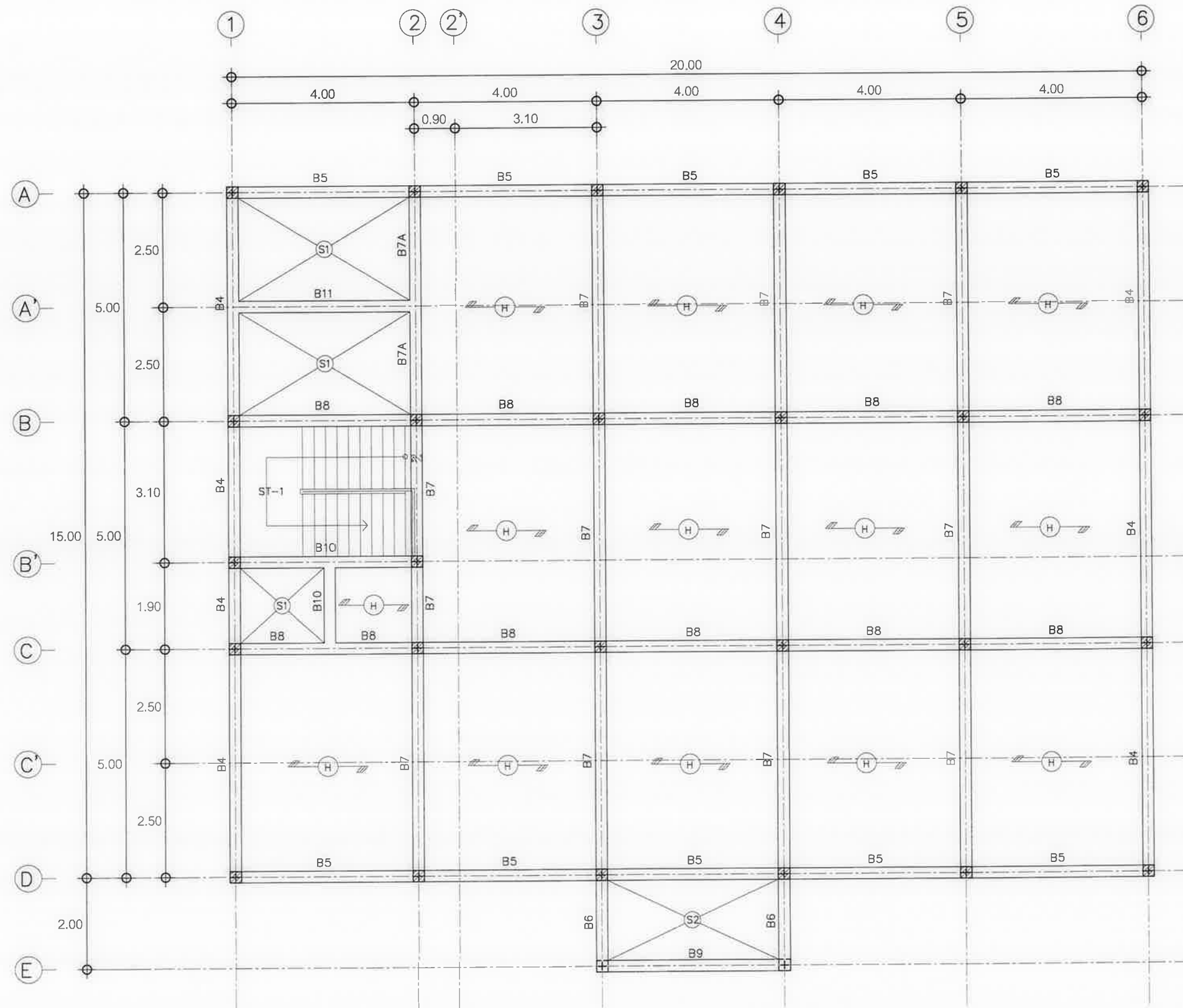
แบบแปลนคานและพื้นชั้น 2 มาตราส่วน 1:100
