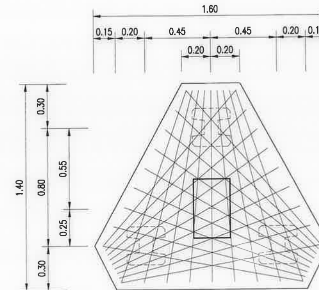
แปลนขยายฐานราก F3 SCALE 1:25
