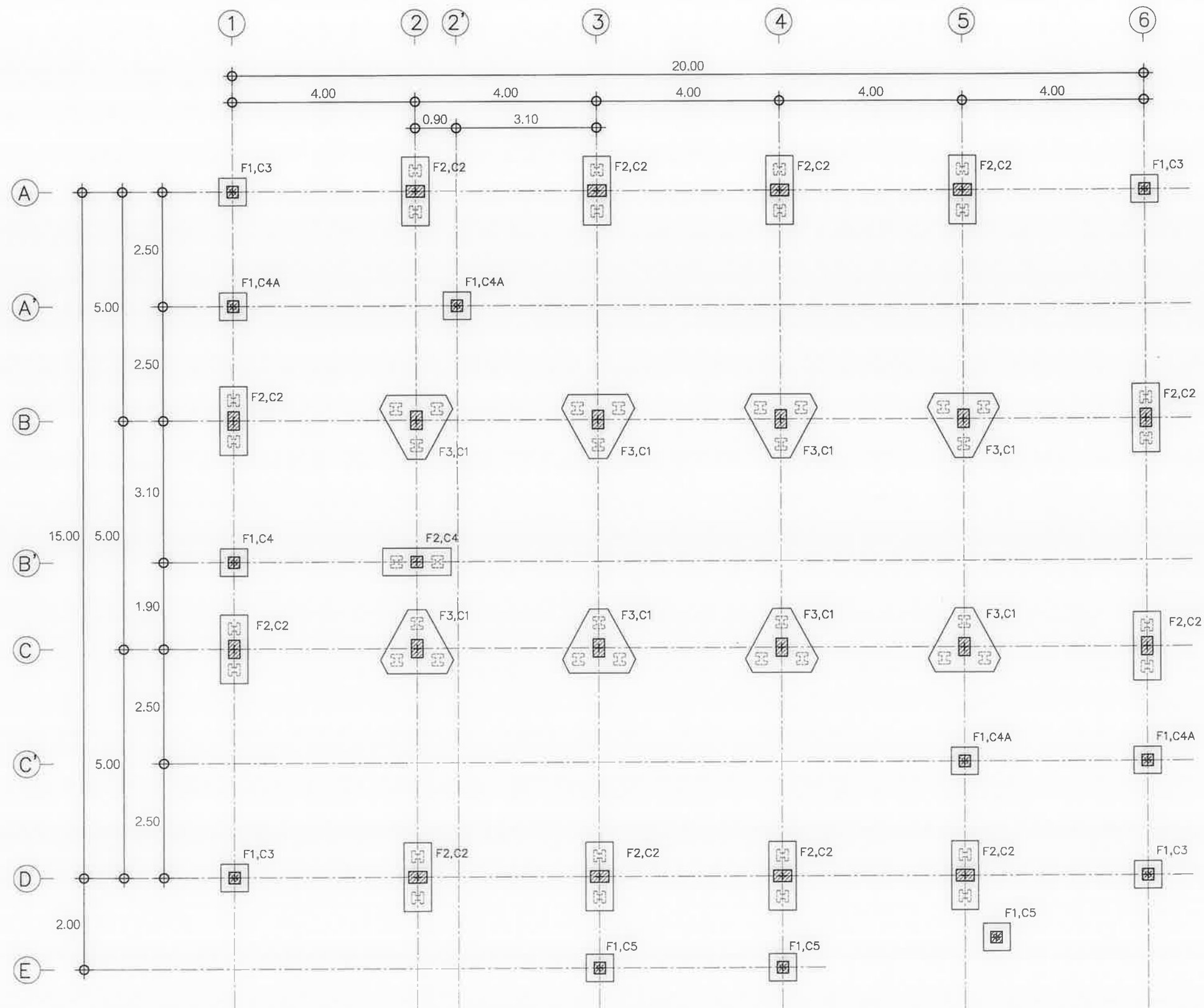
แบบแปลนฐานราก มาตราส่วน 1:100
