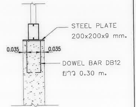
แบบขยาย SUPPORT หัวเสา SCALE 1:20
