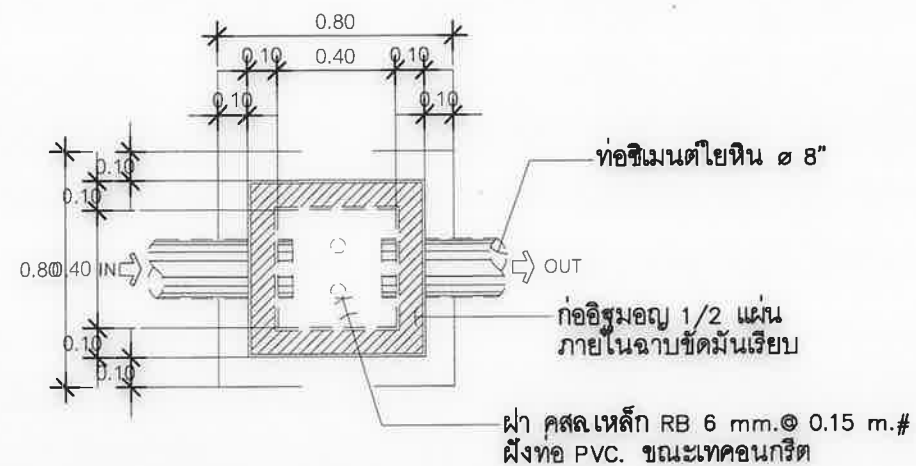
แปลนขยายบ่อพักน้ำทิ้ง มาตราส่วน 1 : 25
