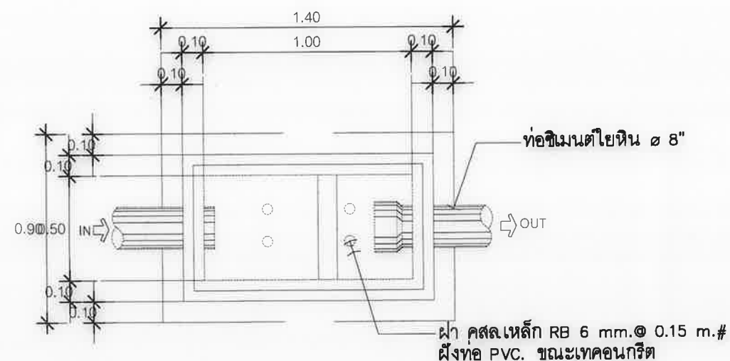
แปลนขยายบ่อดักขยะ-ไขมัน มาตราส่วน 1 : 25
