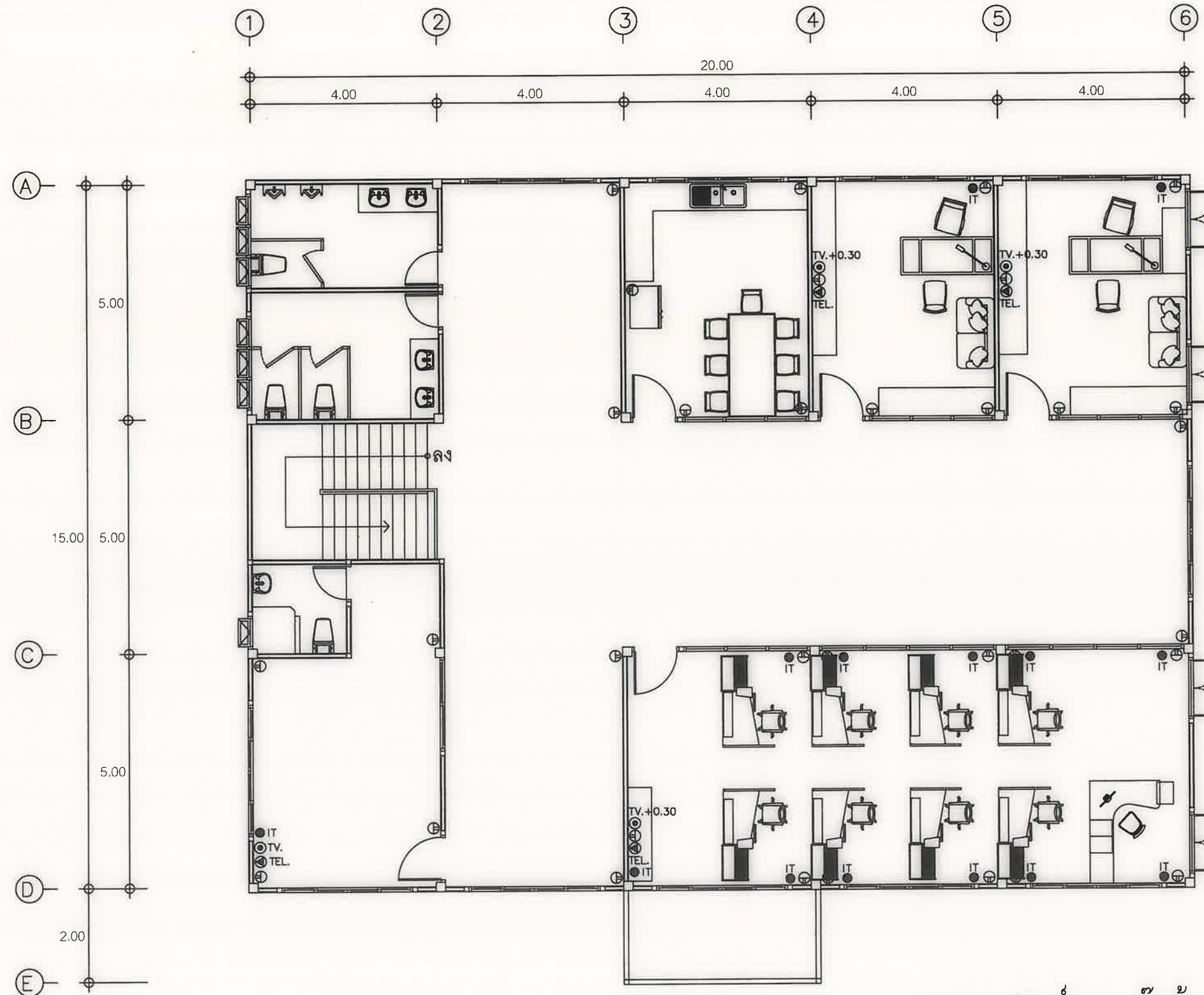
แปลนลิฟท์และปลั๊กชั้น 2 มาตราส่วน 1 : 100
