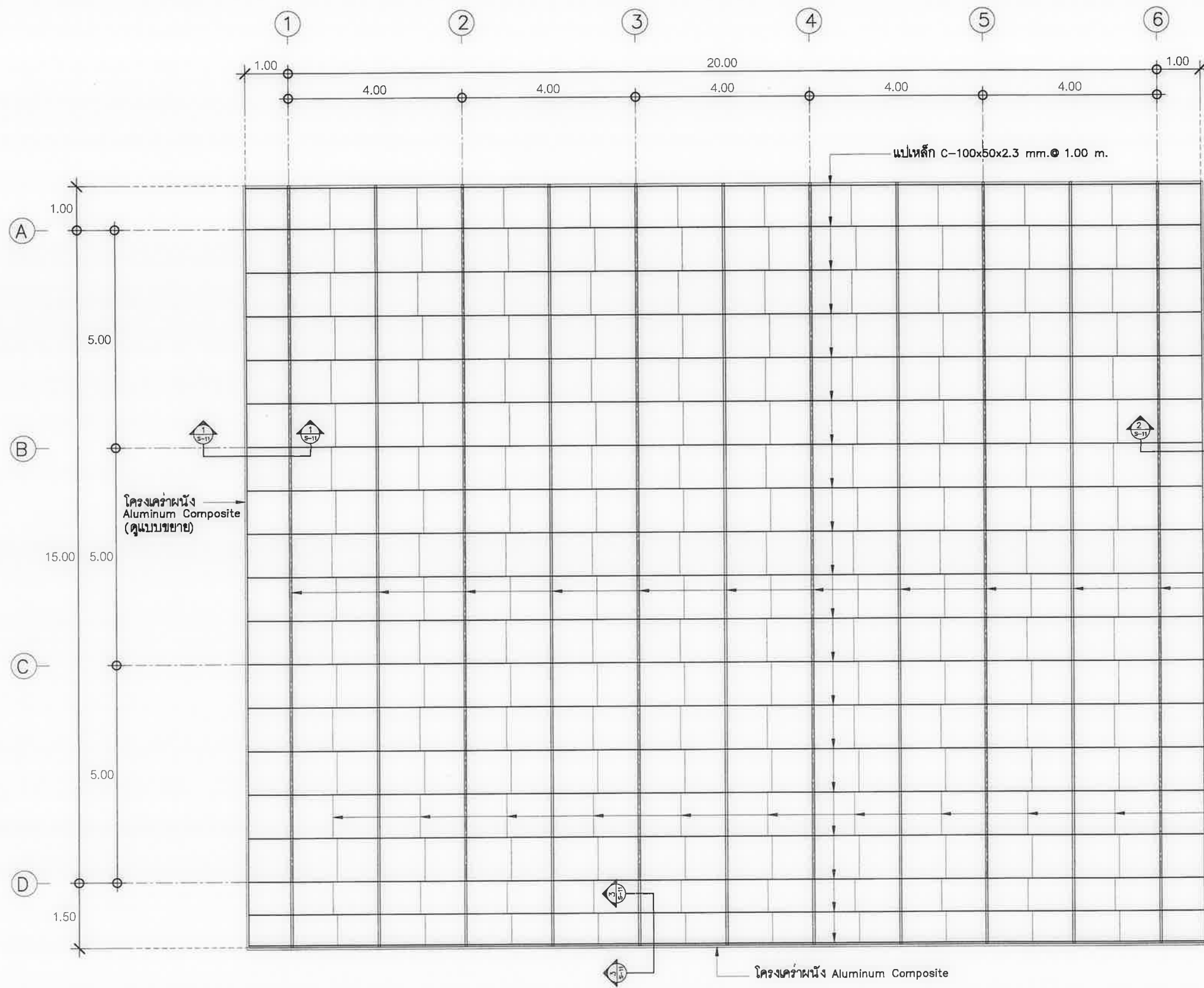
แบบแปลนโครงสร้างหลังคา มาตราส่วน 1:100
