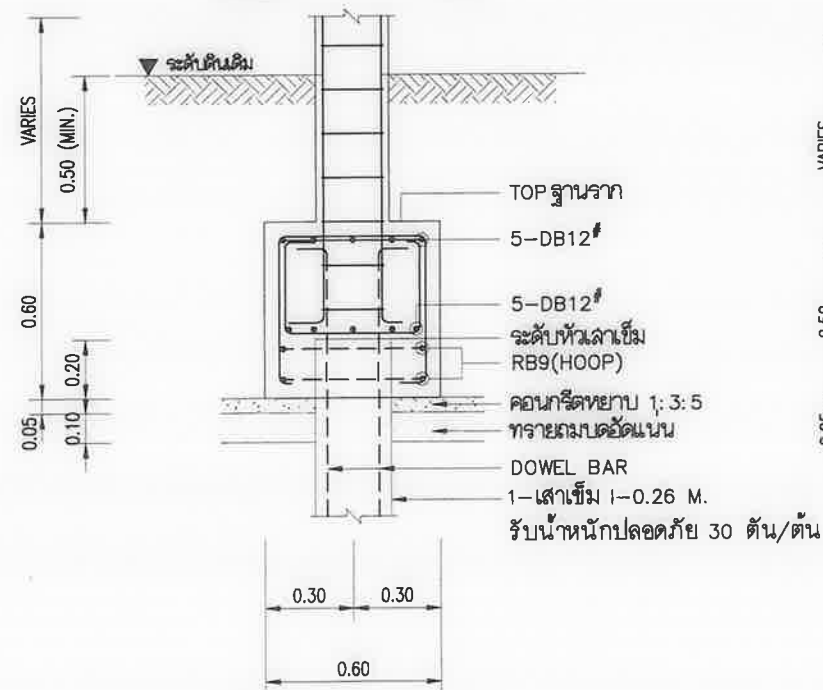
รูปตัดขยายฐานราก F1 SCALE 1:25
