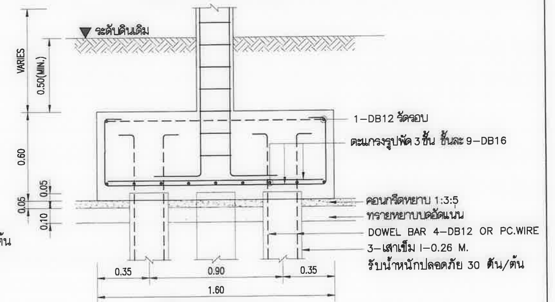
รูปตัดขยายฐานราก F3 SCALE 1:25
