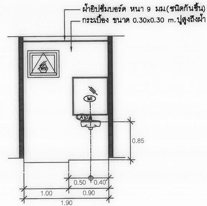
รูปตัด 8 มาตราส่วน 1:50
