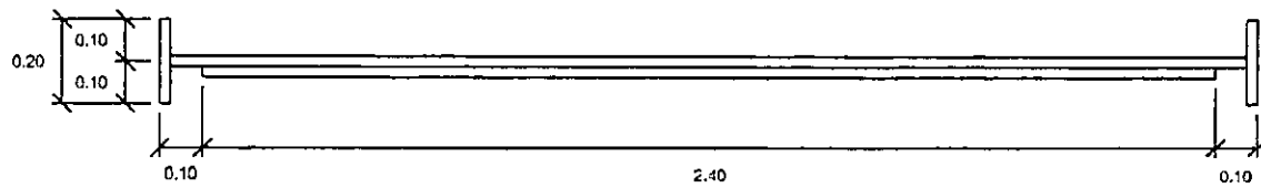
แปลน 1 : 50
