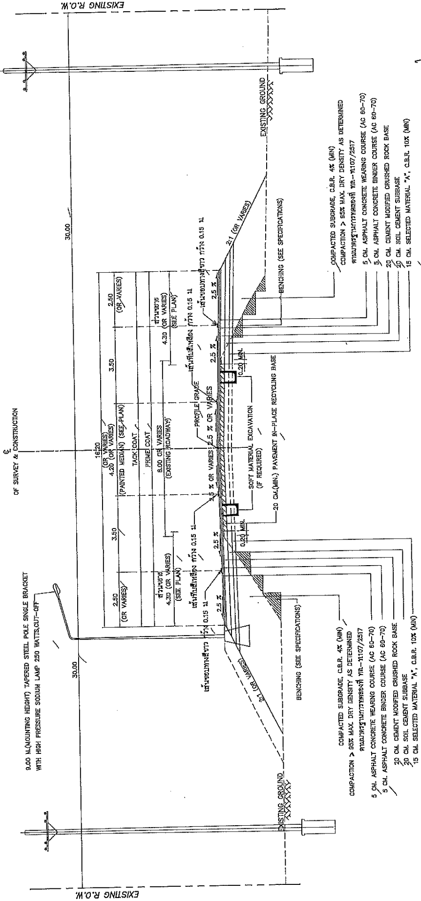
TYPICAL CROSS SECTION (หลังการปรับปรุง) กม.51+795.000 - กม.51+865.000 RT.L.T. กม.52+225.000 - กม.52+345.000 RT.L.T.
