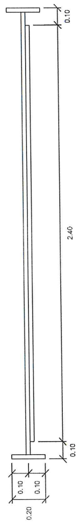
รูปด้านข้าง 1 : 50
