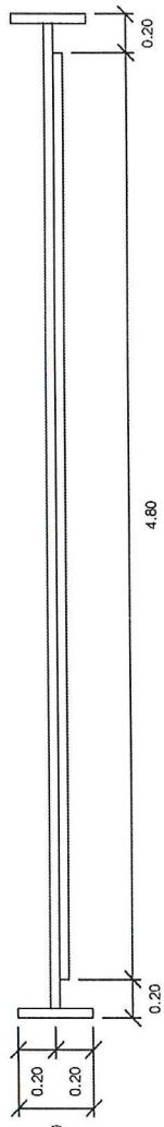
แปลน 1 : 25
