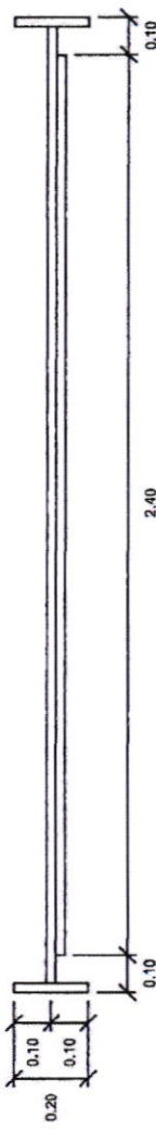
รูปด้านหน้า 1 : 50
