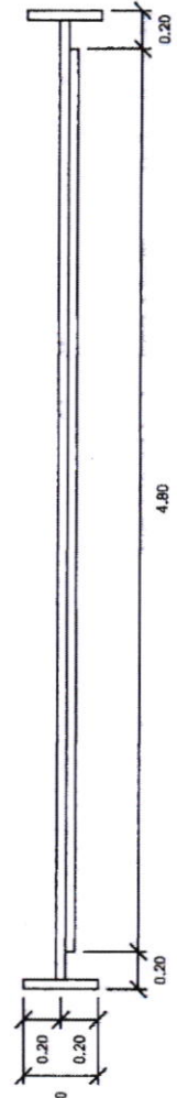
รูปด้านข้าง 1 : 25
