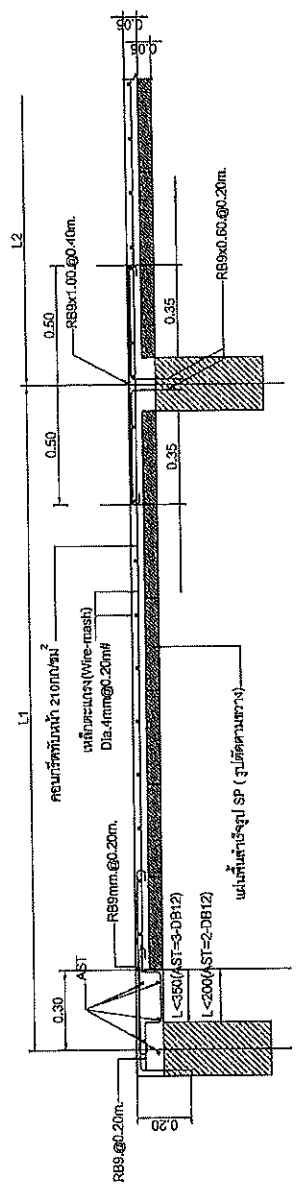
แบบขยายพื้น (PS) (รูปตัดกรณีมีดช่องที่ขาด) SCALE 1/20
