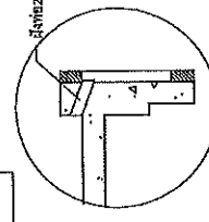
แบบขยาย OVERFLOW ขนาดฐาน 1:25
