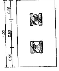
แปลนขยายฐานราก F2 SCALE 1/25
