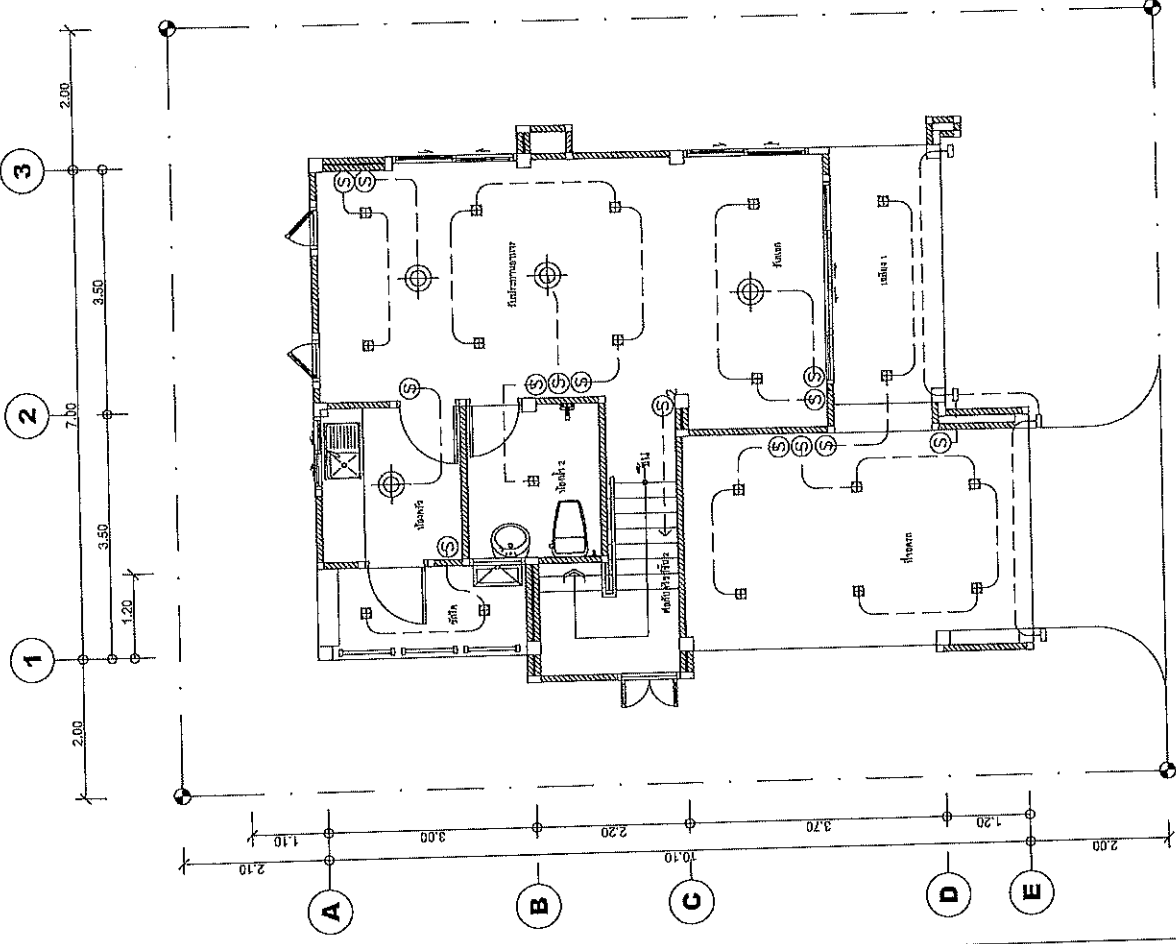
แปลนไฟฟ้าแสงสว่างชั้น 1 ขนาดส่วน 1:75
