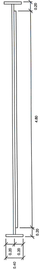
รูปด้านหน้า 1 : 25
