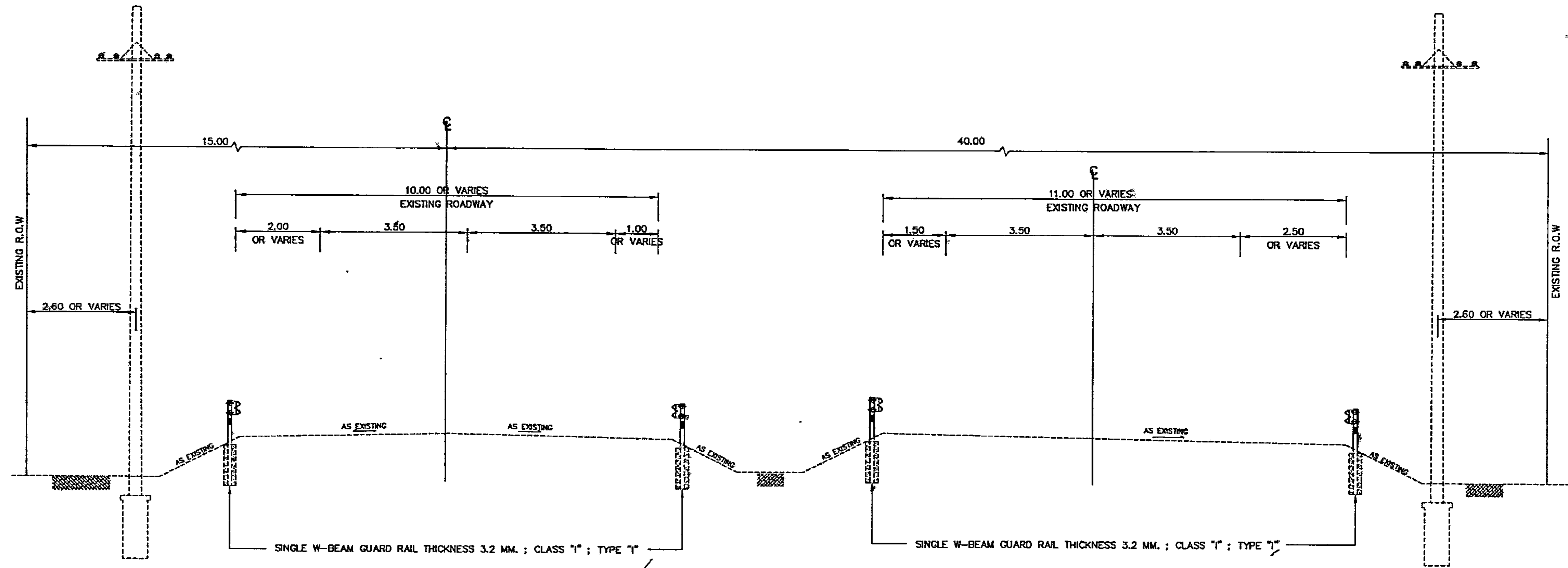
TYPICAL CROSS SECTION SCALE 1:100 กม.257+744 - กม.260+462 (เป็นช่วงๆ)
