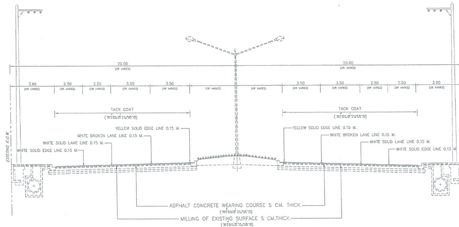
TYPICAL CROSS SECTION ทล.402 ระหว่าง กม.36+694 - กม.36+925 (ก่อนปรับปรุง) SCALE 1:200
