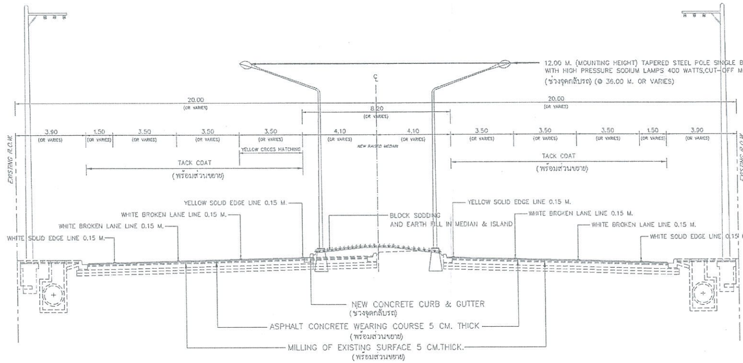
TYPICAL CROSS SECTION ทล.402 ระหว่าง กม.36+194 - กม.36+694 (ก่อนปรับปรุง) SCALE 1:200
