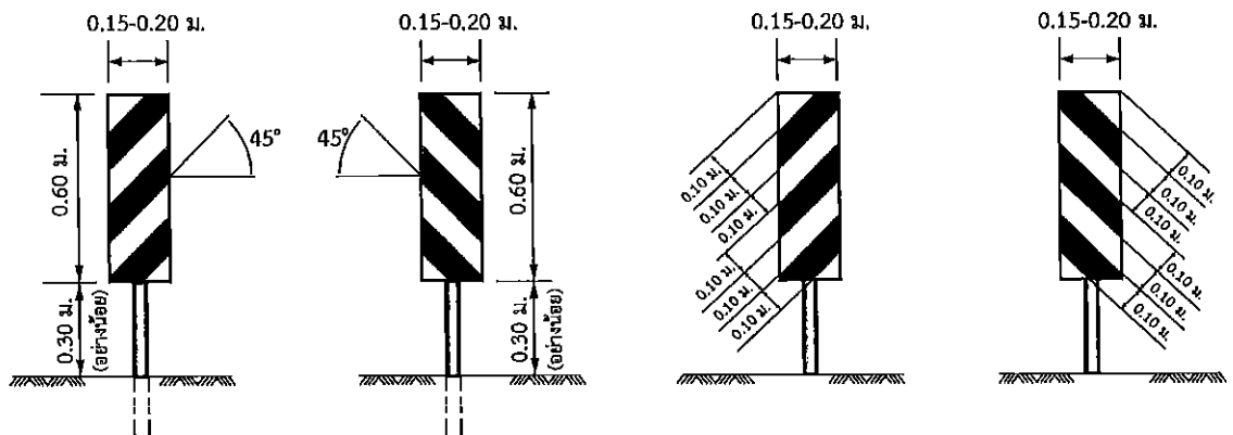
แผงตั้งชนิดวางบนพื้น
