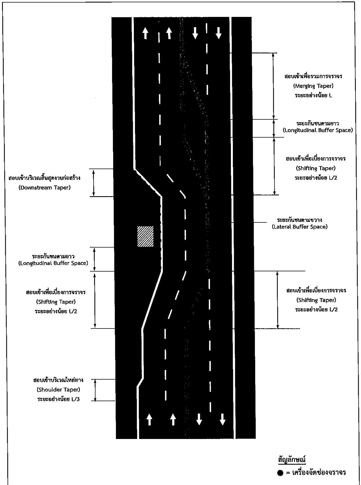
รูปที่ 1-2 ระยะสอเข้า (Taper Length)
