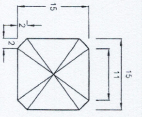
ภาพแสดง มุมมองจากด้านบนอุปกรณ์เสาสลักหน้าทางยาวพารา
