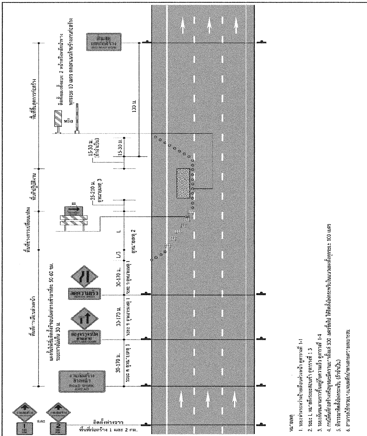
รูปที่ 4-4 การติดตั้งป้ายในงานก่อสร้าง/งานบูรณะ บริเวณช่องจราจรซ้าย สำหรับทางหลวงหลายช่องจราจร
