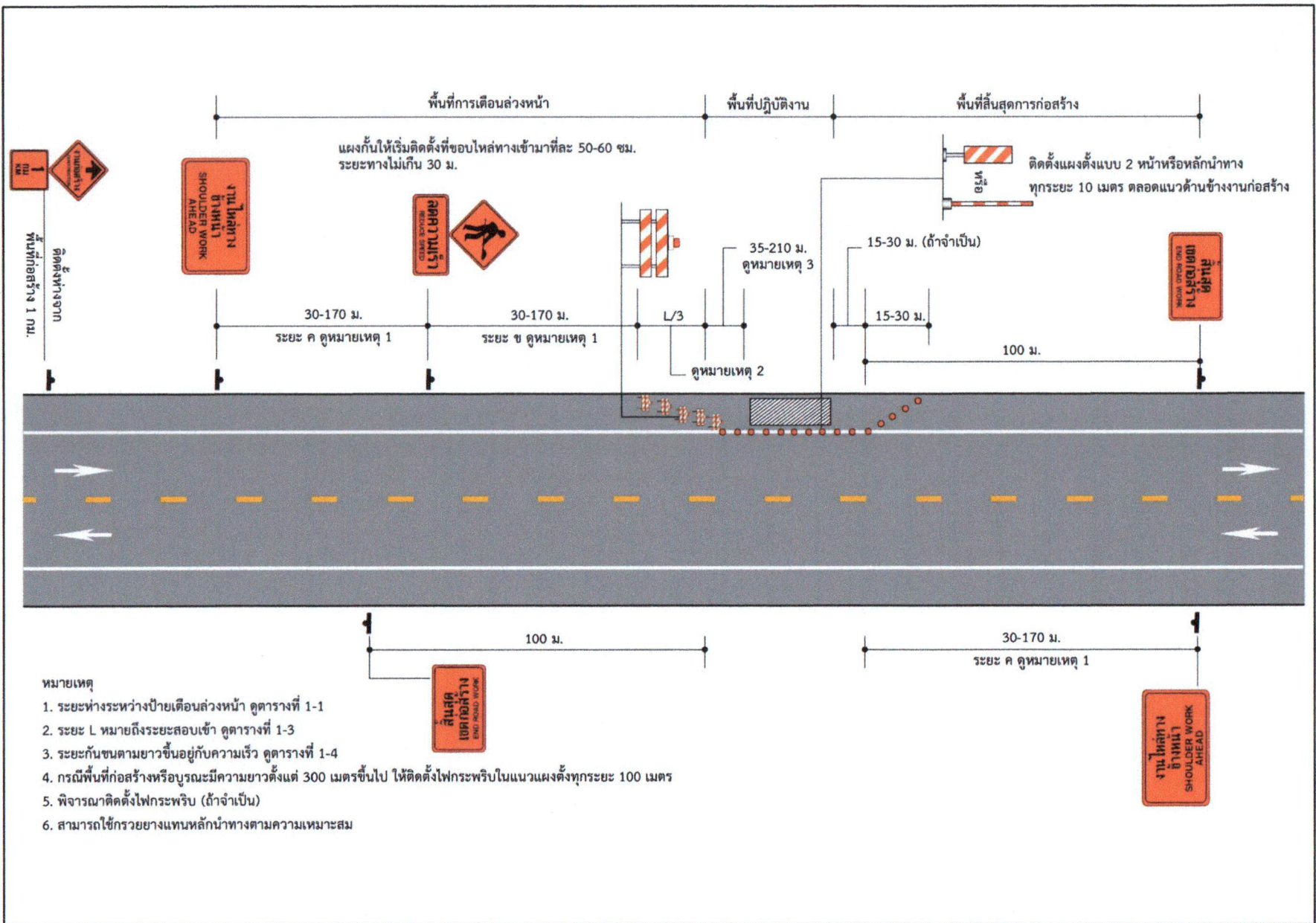
รูปที่ 4-1 การติดตั้งป้ายในงานก่อสร้าง/งานบูรณะ บริเวณไหล่ทาง สำหรับทางหลวง 2 ช่องจราจร
