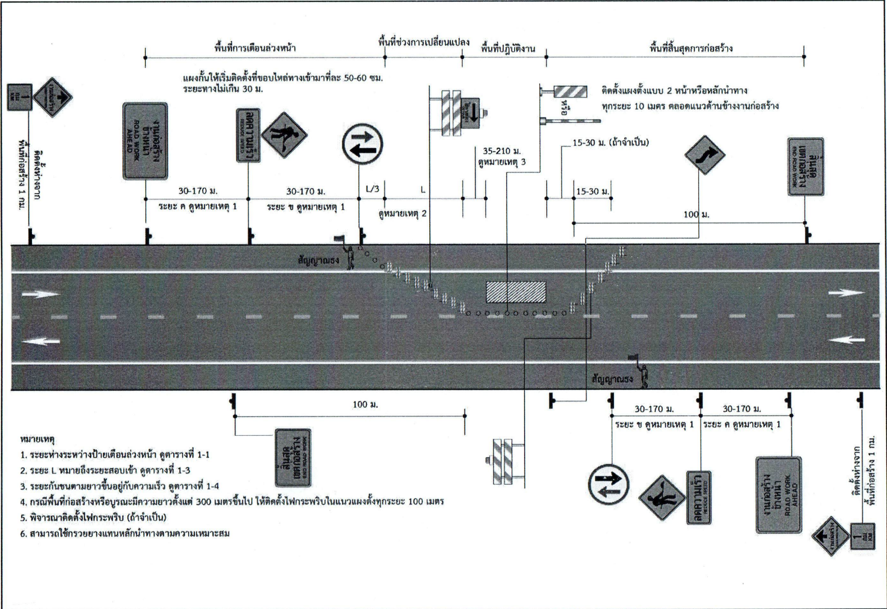
รูปที่ 4-3 การติดตั้งป้ายในงานก่อสร้าง/งานบูรณะ บริเวณช่องจราจรซ้าย สำหรับทางหลวง 2 ช่องจราจร
