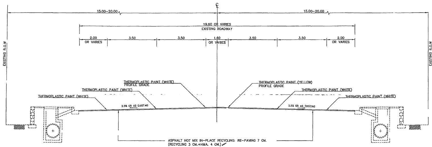
TYPICAL CROSS SECTION SCALE 1:100 กม. 33+198 / กม. 35+200
