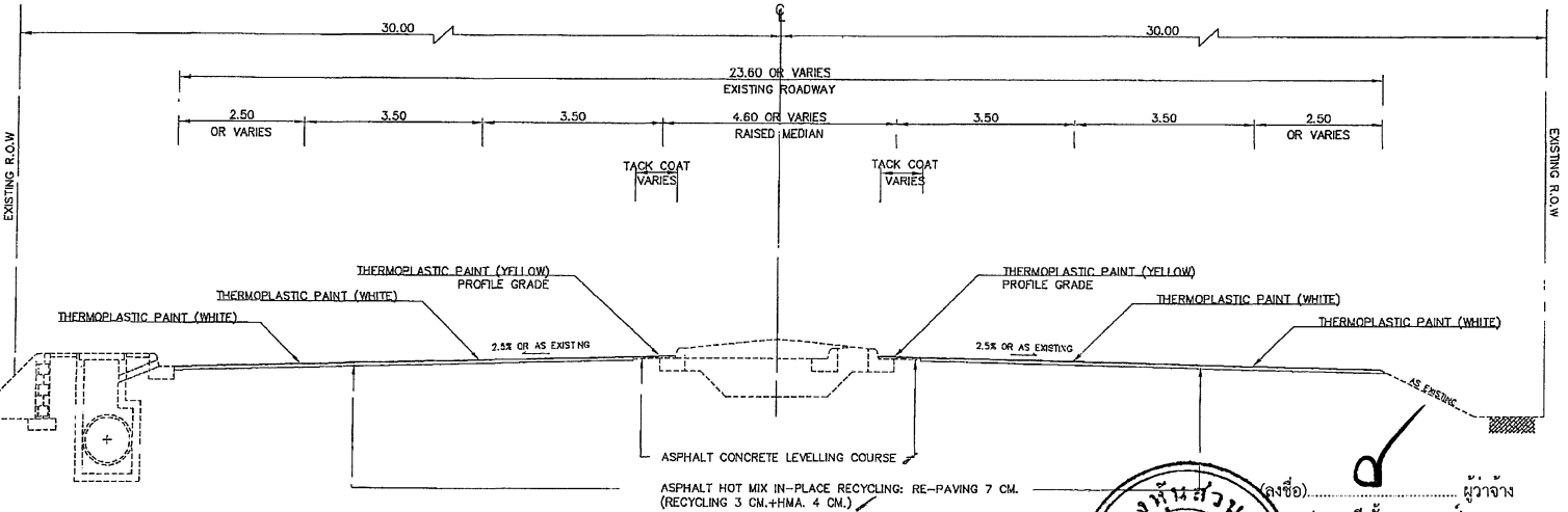
TYPICAL CROSS SECTION (II) SCALE 1:100 กม. 63+165 - กม. 64+432 (เป็นตอนๆ)
