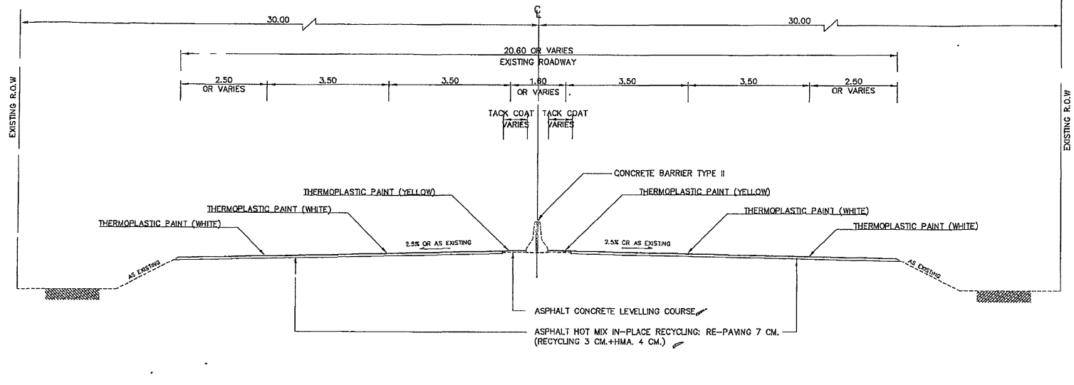
TYPICAL CROSS SECTION (I) SCALE 1:100 กม. 60+450 - กม. 61+810 (เป็นตอนๆ)
