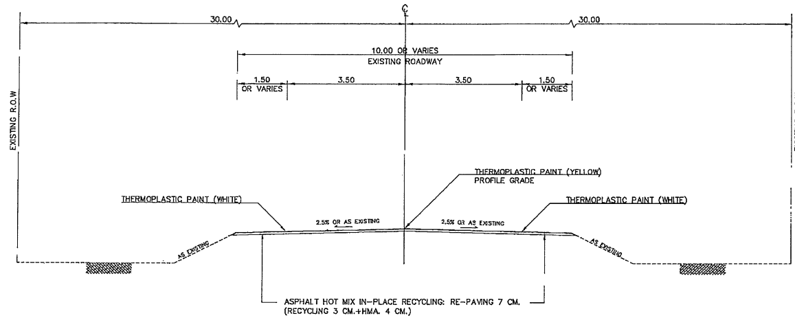
TYPICAL CROSS SECTION SCALE 1:100 กม 26+615 - กม 42+540 (เป็นตอนๆ)
