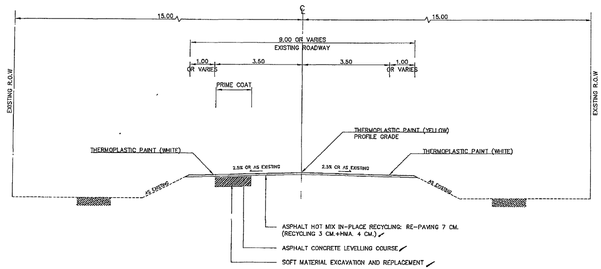
TYPICAL CROSS SECTION SCALE 1:100 กม. 42+800 - กม. 52+100 (เป็นตอนๆ)
