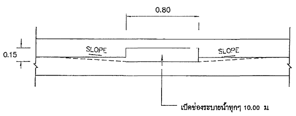
DETAIL ช่องระบายน้ำบริเวณขกโค้ง NOT TO SCALE
