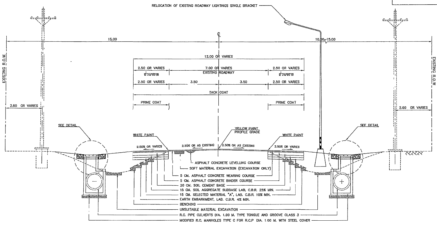
TYPICAL CROSS SECTION 2 SCALE 1:100 กม.5+065- กม.5+100 และ กม.5+300- กม.5+410 (เป็นตอนๆ)
