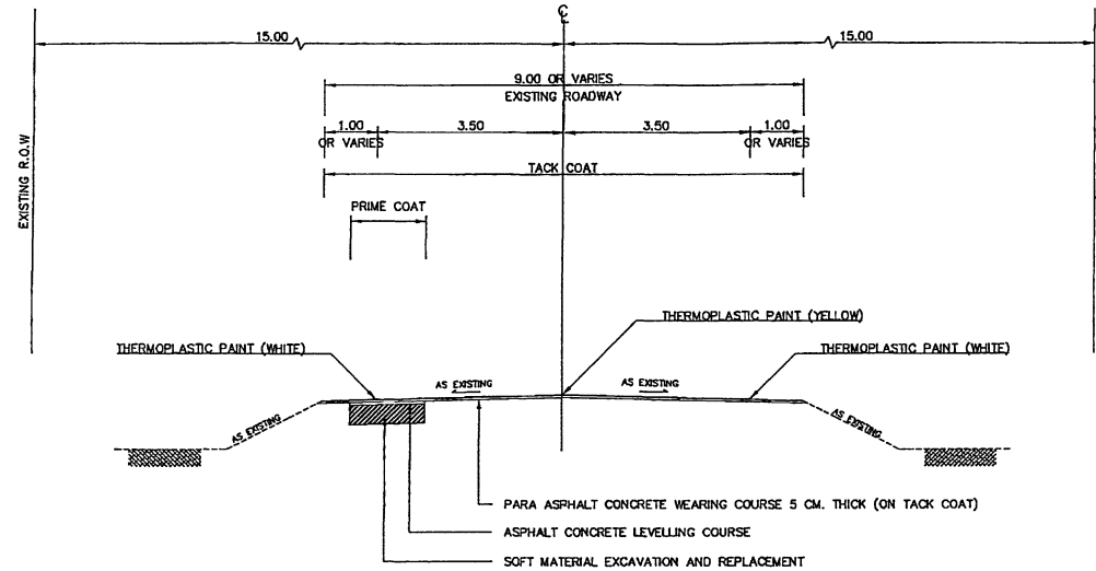
TYPICAL CROSS SECTION SCALE 1:100 กม.5+814 - กม.8+281 และ กม.15+360 - กม.16+300
