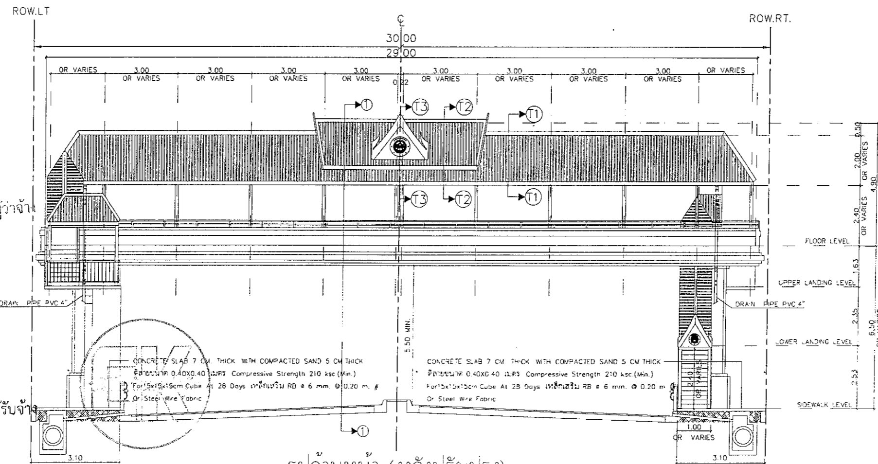
รูปด้านหน้า (หลังปรับปรุง) SCALE 1:150
