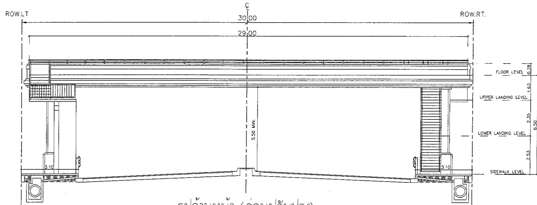
รูปด้านหน้า (ก่อนปรับปรุง) SCALE 1:150
