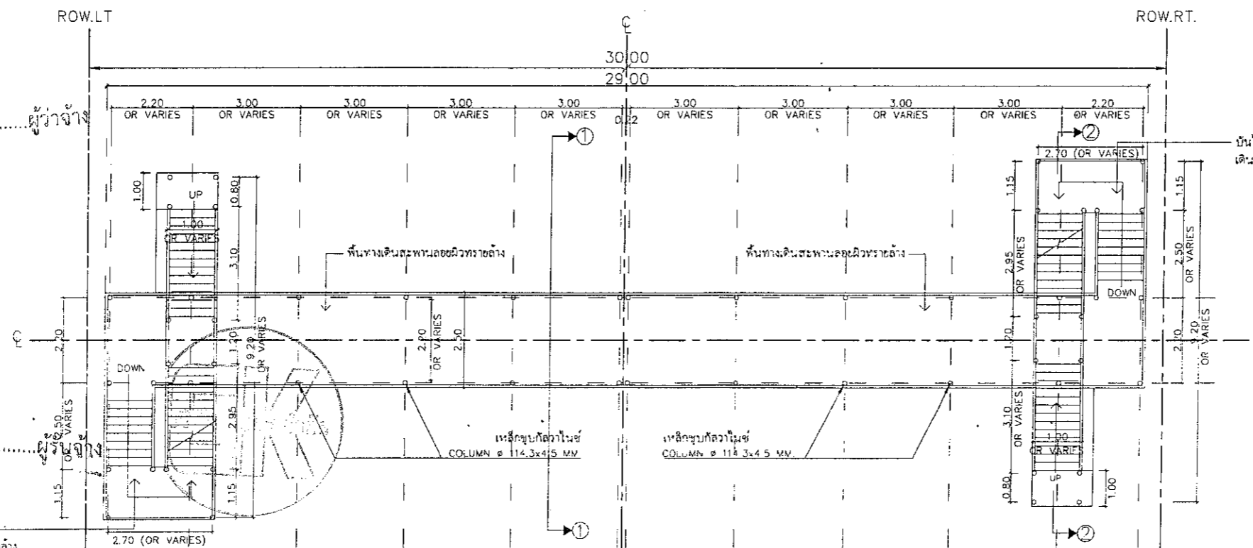
รูปแปลน (หลังปรับปรุง) SCALE 1:150
