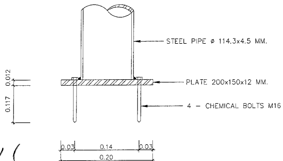
ผู้ว่าจ้าง STEEL PLATE DETAILS
