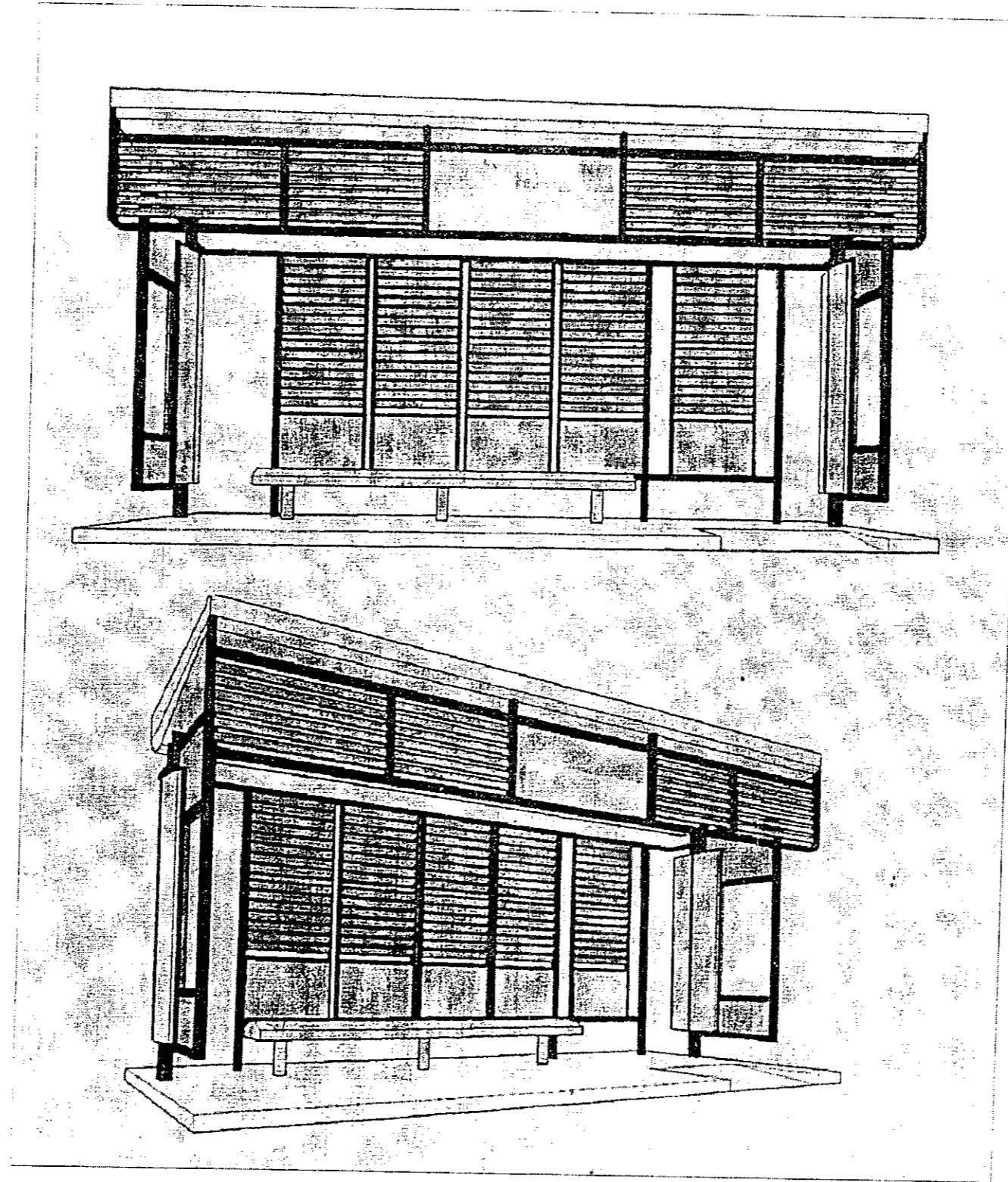
แบบแปลนป้ายรถเมล์แบบที่ ๕ (แบบปรับปรุง) BUS STOP SHELTER TYPE "E" MODIFIED 2020-1
