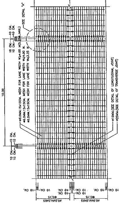
รูปที่ 2 การเสริมเหล็กคานเสริมแรง wire mesh กันรั่วกันน้ำคอนกรีตหนา 25 ซม.
