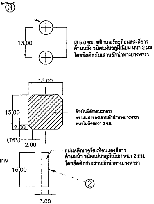
ภาพแสดง ภาพตัด B-B และรายละเอียดสติกเกอร์
