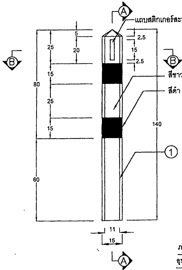
ภาพแสดง มุมมองจากด้านหน้า รูปกรณ์เสาหลักนำทางยางพารา
