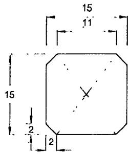
ภาพแสดง เสาหลักนำทางยางพารา (ด้านบน)
