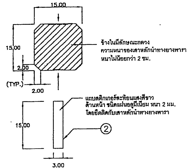
ภาพแสดง ภาพตัด B - B และรายละเอียดสติกเกอร์สะท้อนแสง
