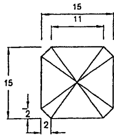
ภาพแสดง มุมมองจากด้านบนรูปกรณ์เสาหลักนำทางยางพารา
