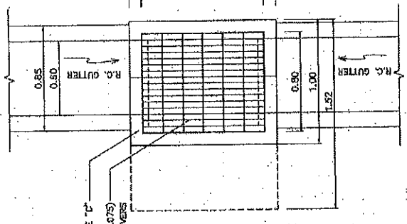
R.C. MANHOLE TYPE "T"
