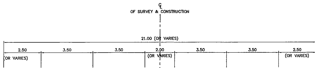
รูปตัดทั่วไปก่อนดำเนินการปรับปรุง กม.17+814 - กม.18+697
