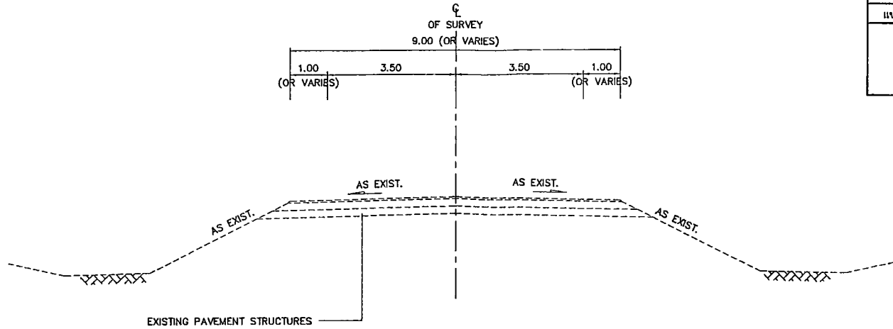
รูปตัดทั่วไปก่อนดำเนินการปรับปรุง กม 9+948 - กม 10+623
