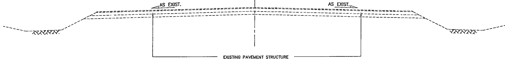
รูปตัดทั่วไปก่อนดำเนินการปรับปรุง กม.17+814 - กม.18+697
