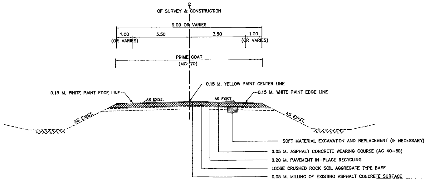
รูปตัดทั่วไปก่อนดำเนินการปรับปรุง กม 9+948 - กม 10+623
