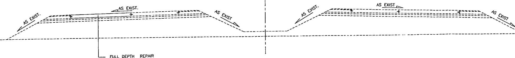
รูปตัดทั่วไปหลังดำเนินการปรับปรุง กม.135+260 - กม.154+000 (เป็นแห่งๆ)
