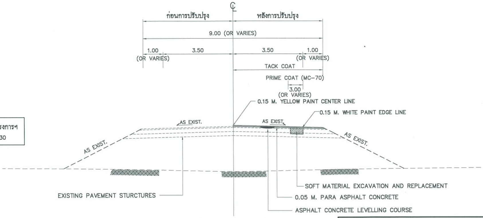
TYPICAL CROSS SECTION กม.2+930 - กม.6+270 (เป็นตอน ๆ)
