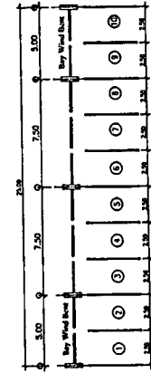
แปลน Zone B
