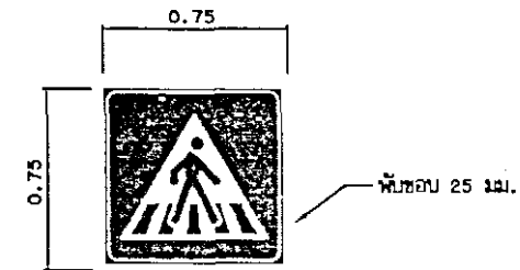
แบบขยายป้ายเตือนทางข้าม (แบบพับขอบ)
