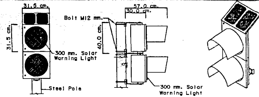
แบบขยายสัญญาณไฟกระพริบ แบบ 2 หัว
