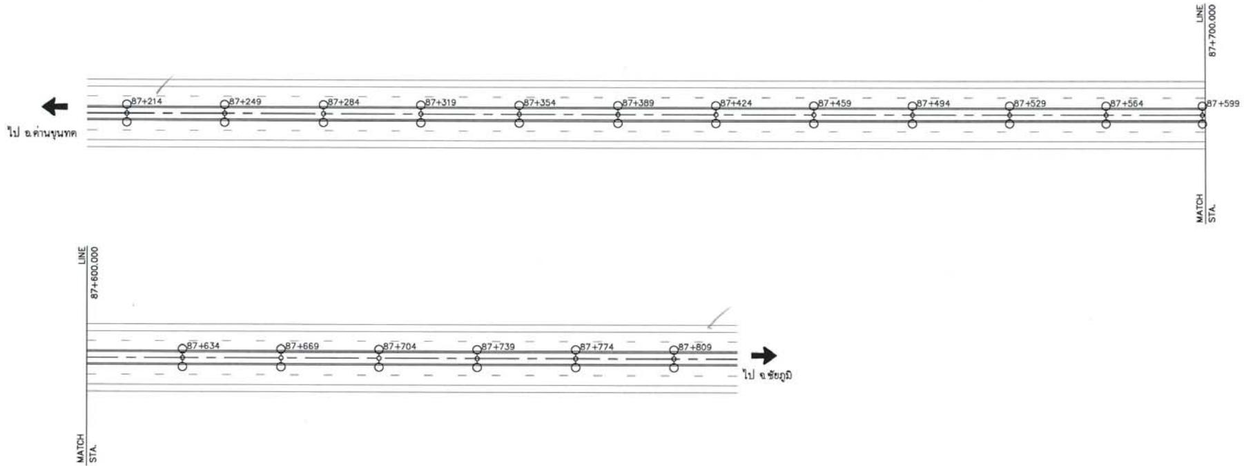
แบบแนะนำตำแหน่งติดตั้งไฟฟ้าแสงสว่าง NOT TO SCALE
