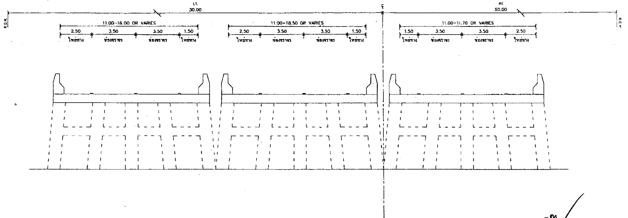
รูปตัดก่อนดำเนินการ
