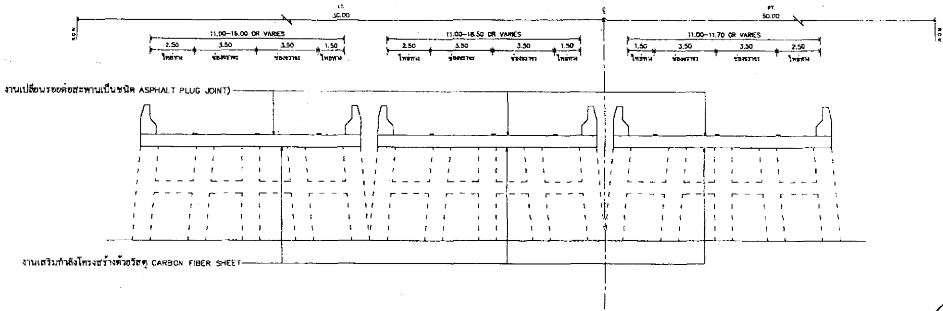
รูปตัดหลังดำเนินการ
