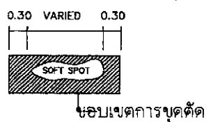
รูปแสดงการแก้ไขจุดอ่อนตัว (SOFT SPOT)
