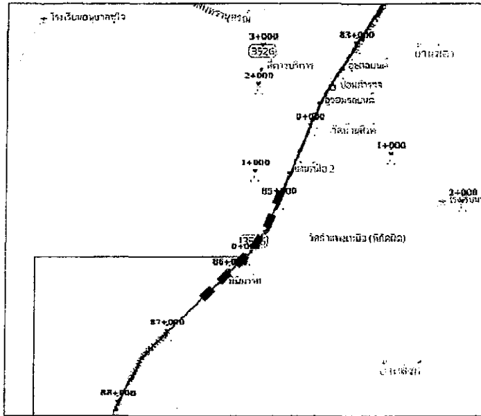
ตำแหน่งโครงการ ระหว่าง กม.85+000 - กม.86+450 LT.
