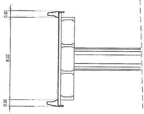
EXISTING CROSS SECTION STA. 44+000
