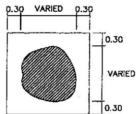
รูปแบบเขตการขุดตัด
