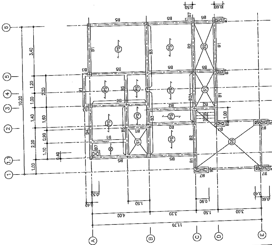
แปลนคานาพื้นชั้น 1 1:100 มาตราส่วน
