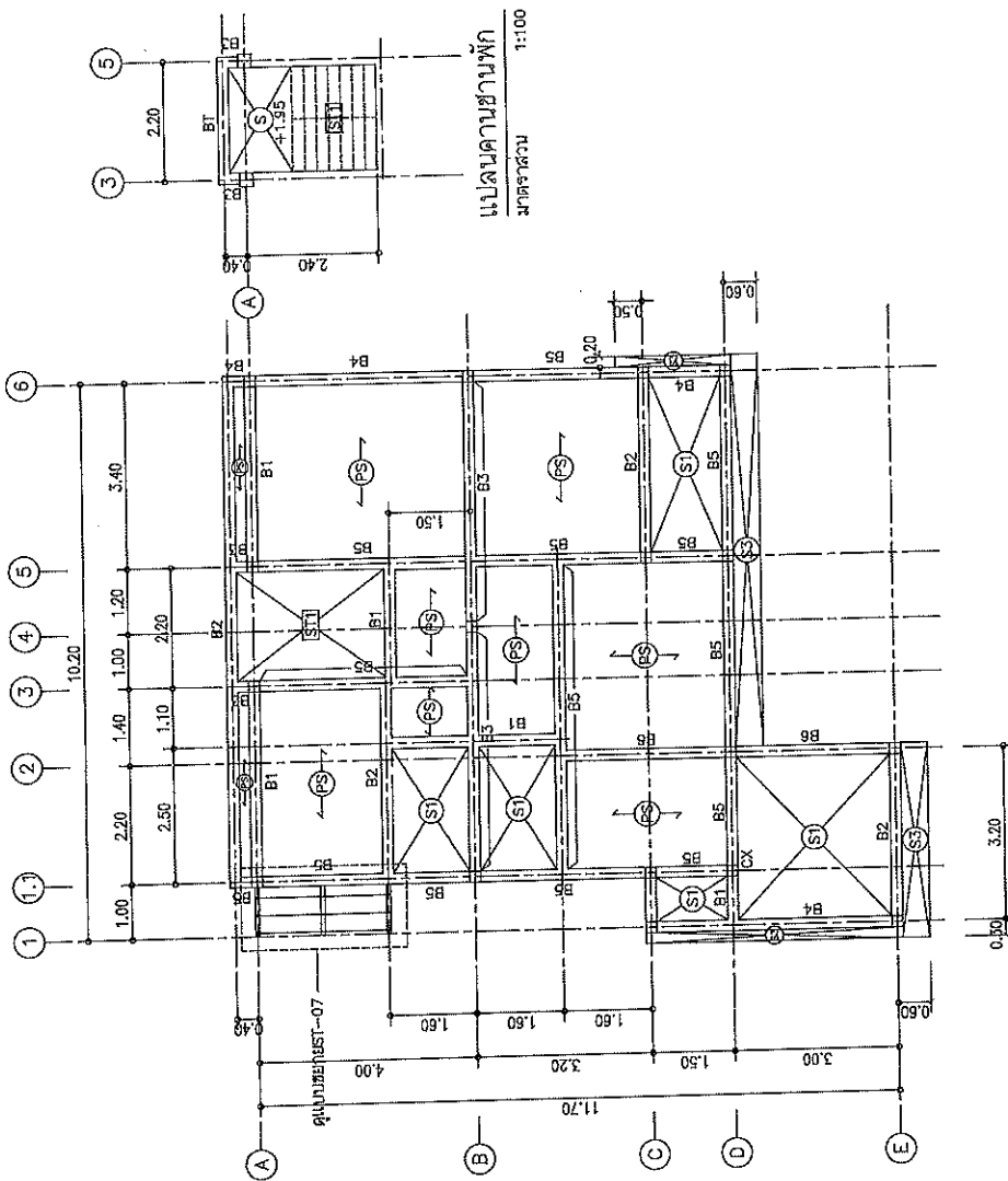
แปลนคานาพื้นชั้น 2 1:100 มาตราส่วน
