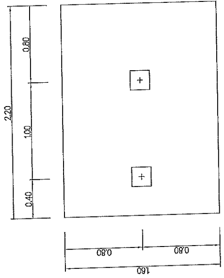
แปลนขยายฐานราก FE มาตราส่วน 1:25
