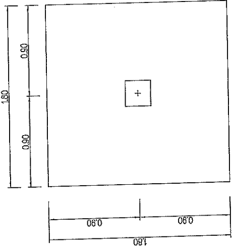
แปลนขยายฐานราก FB มาตรฐาน ขนาดฐาน 1:25
