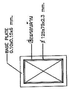
SECTION A - A มาตราส่วน 1:5
