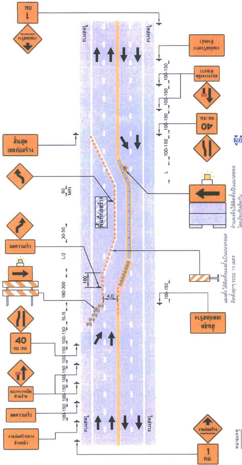
รูปที่ 9-10 แบบป้ายมาตรฐานในงานก่อสร้าง ซุดทางหลวง 4 ช่องจราจร ไม่มีเกาะกลาง ปิดการจราจรหนึ่งทิศทาง
