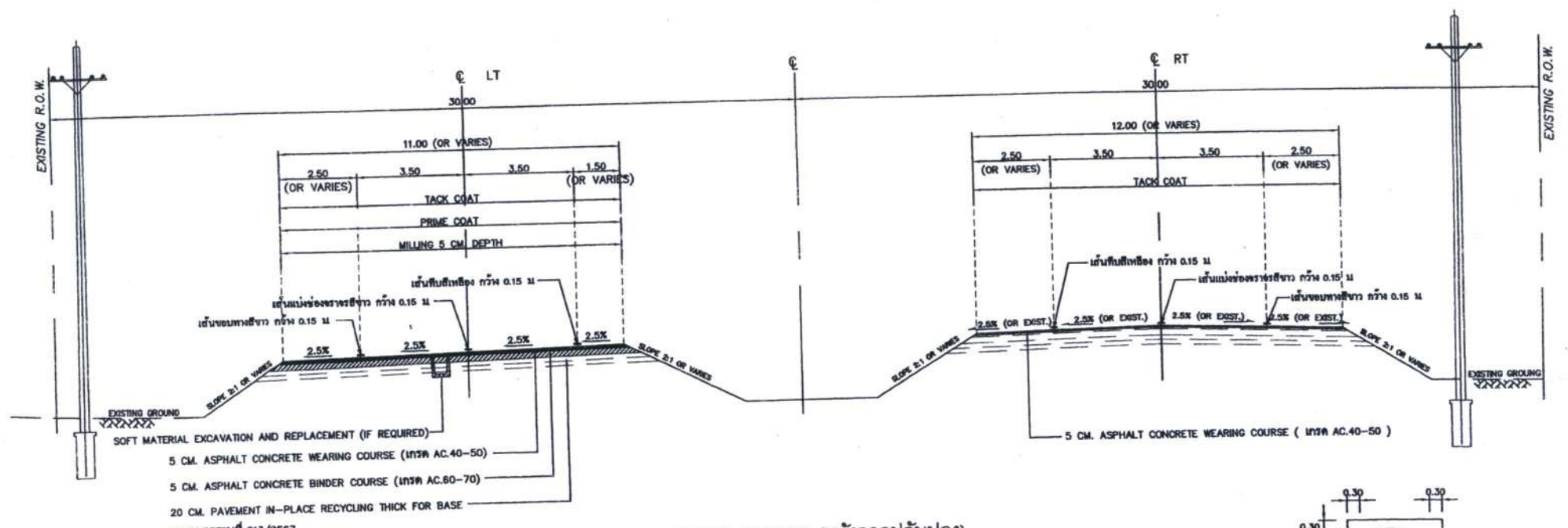
TYPICAL CROSS SECTION (หลังการปรับปรุง) กม.4+550.000 - กม.4+753.000 NOT TO SCALE
