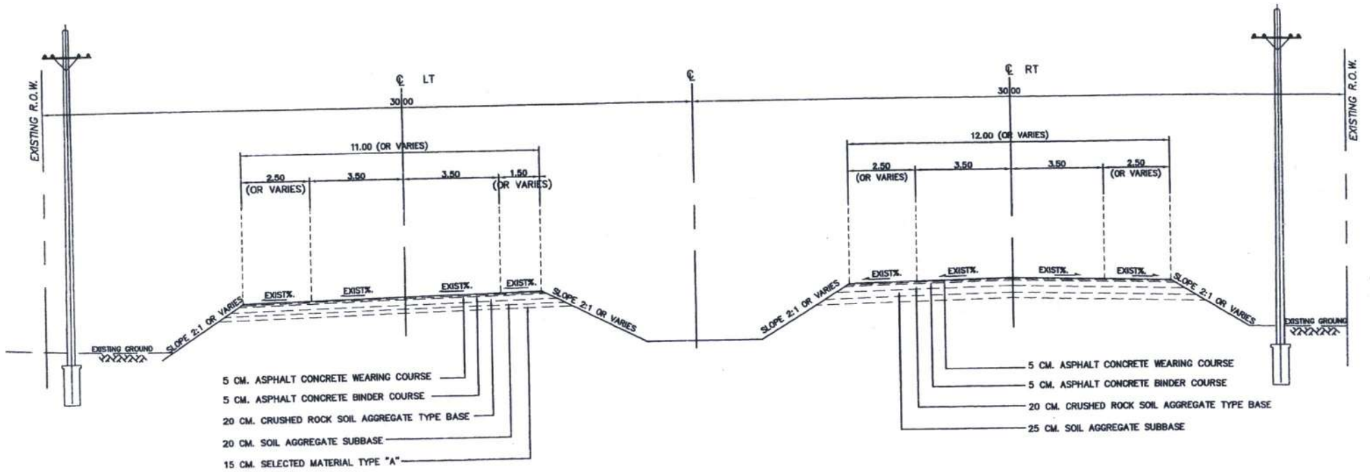
TYPICAL CROSS SECTION (ก่อนการปรับปรุง)
